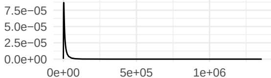
Precision parameter for the beta observation
