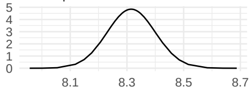
precision parameter for the beta observation
