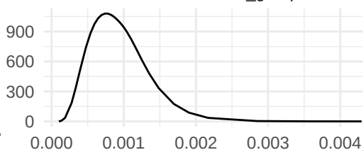
Precision parameter for the beta observations[
