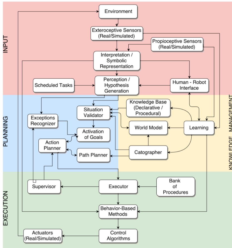
Figura 3.1: Arquitectura general ViRBot del robot Justina.
