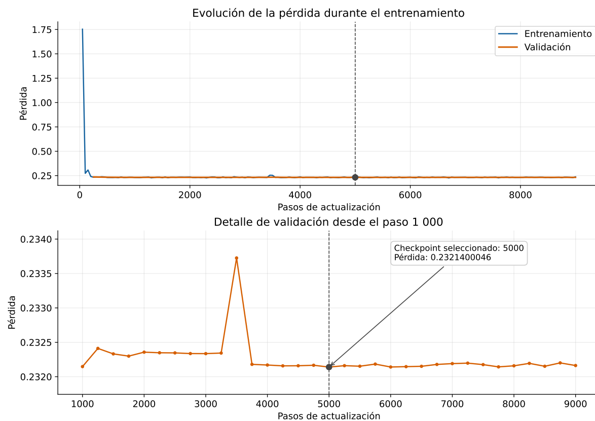
Figura 5.1: Evolución de las pérdidas de entrenamiento y validación durante el ajuste de Qwen2.5-7B mediante QLoRA. La pérdida de entrenamiento se registra cada 50 actualizaciones y la de validación cada 250. Se muestra el historial completo, hasta el paso 9 000. Elaboración propia.
