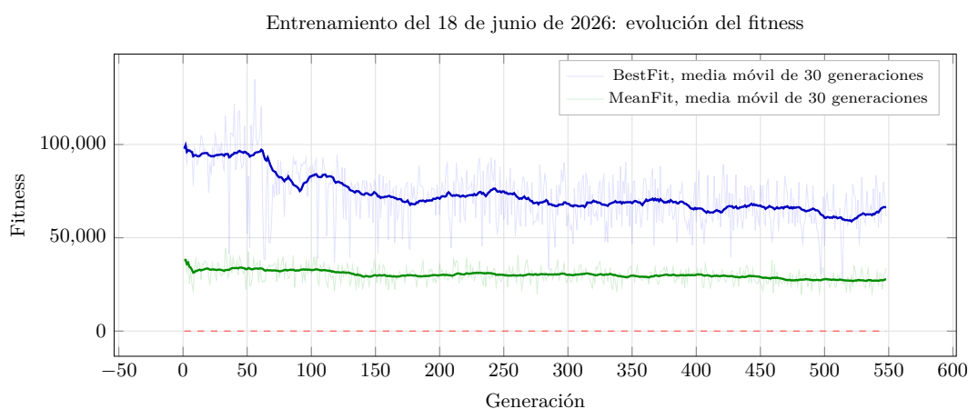
Figura 6.1: Tendencia del fitness en el entrenamiento del 18 de junio de 2026. Fuente: análisis generado a partir de Training_Summary.csv .
