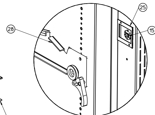
Dettaglio3 Scala 1:3
