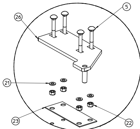
Dettaglio2 Scala 1:4
