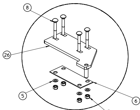
Dettaglio3 Scala 1:5
