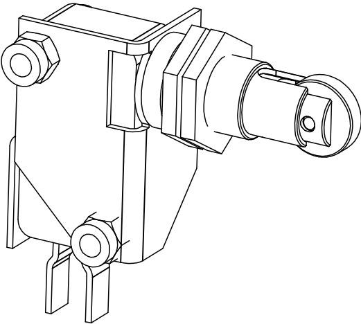
Scala 1.5:1
