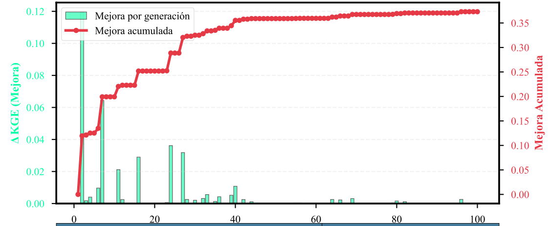
Mejora del Fitness
