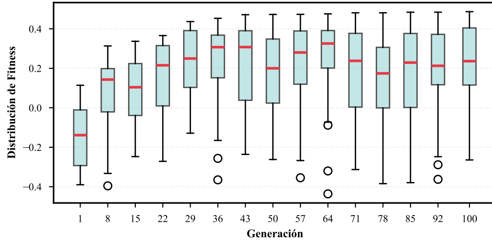
Convergencia del Algoritmo
