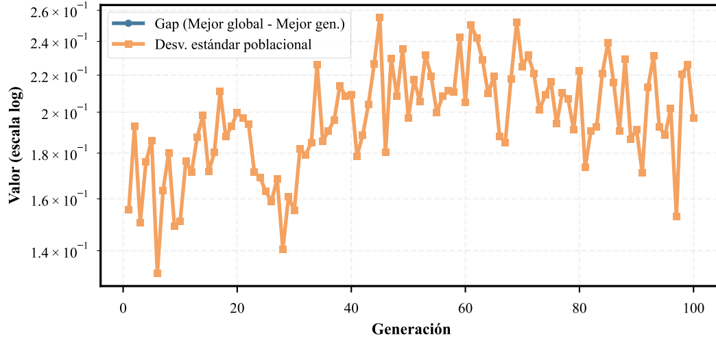
Convergencia del Algoritmo
