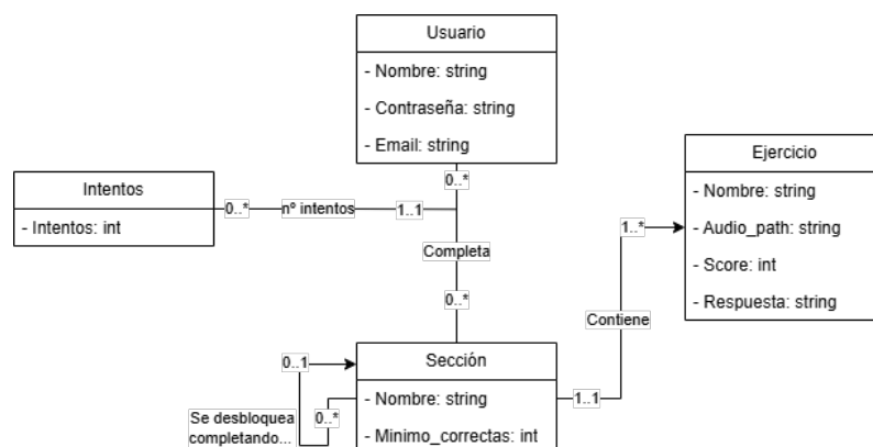
Figura 4.1: Diagrama UML de la Base de Datos.
