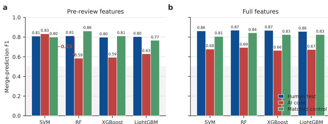
图 1 传统机器学习模型在人类代码、AI 代码与匹配人类对照上的合并预测 F1。a, pre-review 特征；b, 包含审查过程变量的 full 特征。蓝、红、绿分别表示实验二人类 held-out test、AI 代码和匹配人类对照。RF、XGBoost 和 LightGBM 在 AI 侧的 pre-review F1 下降，full 设置下四个模型的 AI F1 均低于两个人类锚点。图中为单次固定划分的点估计，不含误差条。
