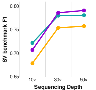
minimap2
