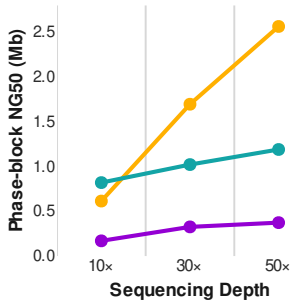
minimap2
