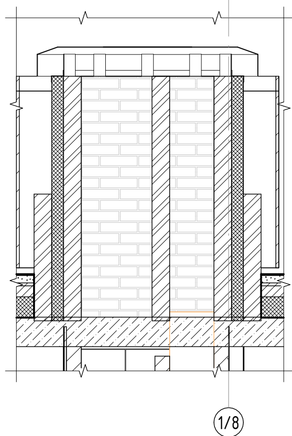
Разрез 8 - 8 ( 1 : 25)
