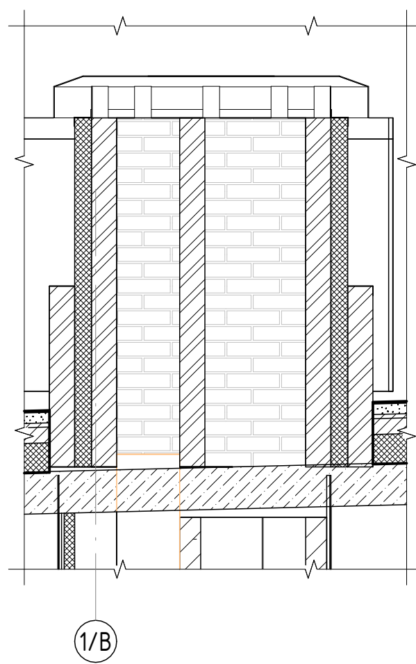
ВШ-9 ( 1 : 25)
