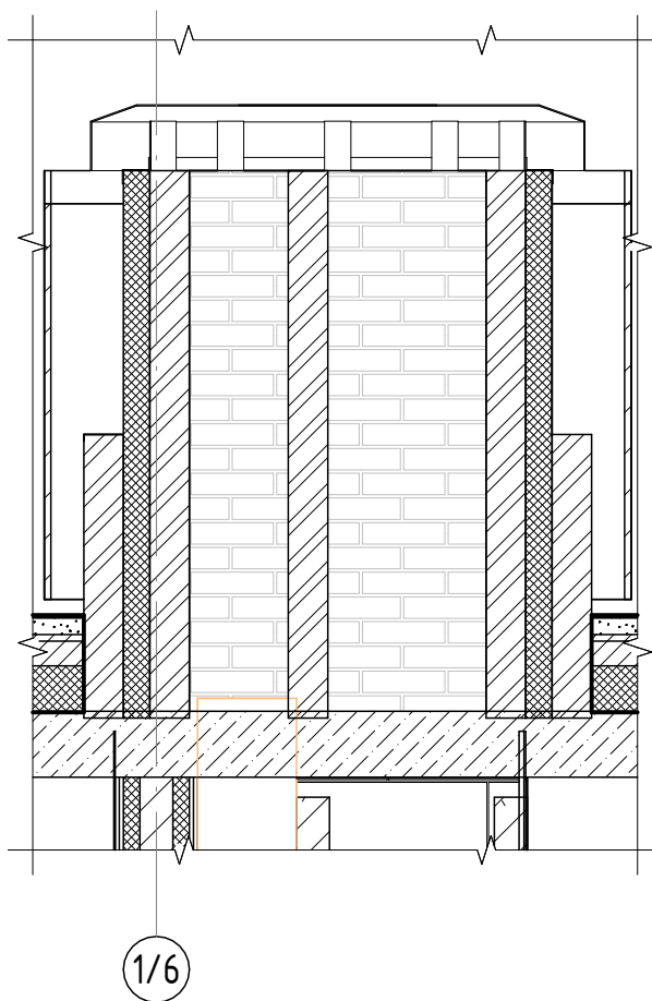
Разрез 6 - 6 ( 1 : 25)
