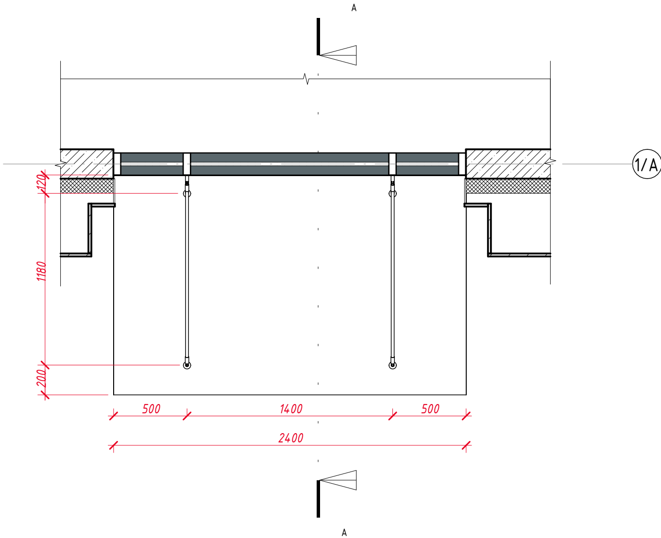
Козырек Ко-1 ( 1 : 25)
