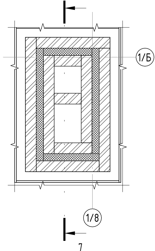
Разрез 7 - 7 ( 1 : 25)
