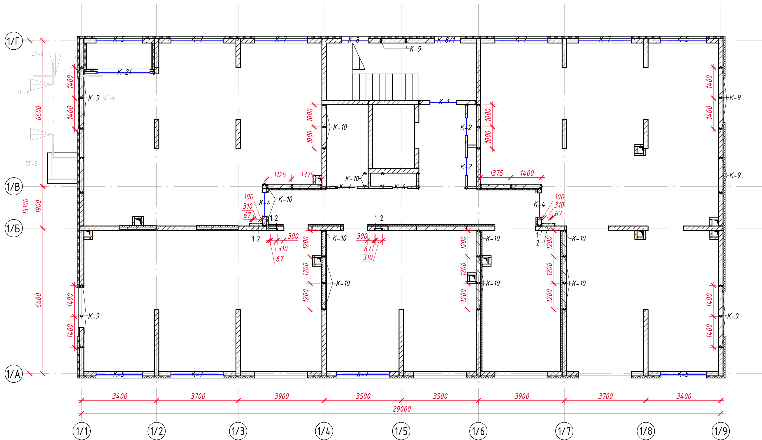
План отверстий и усиления проема 1го этажа на отм. +0,000 ( 1 : 100)
