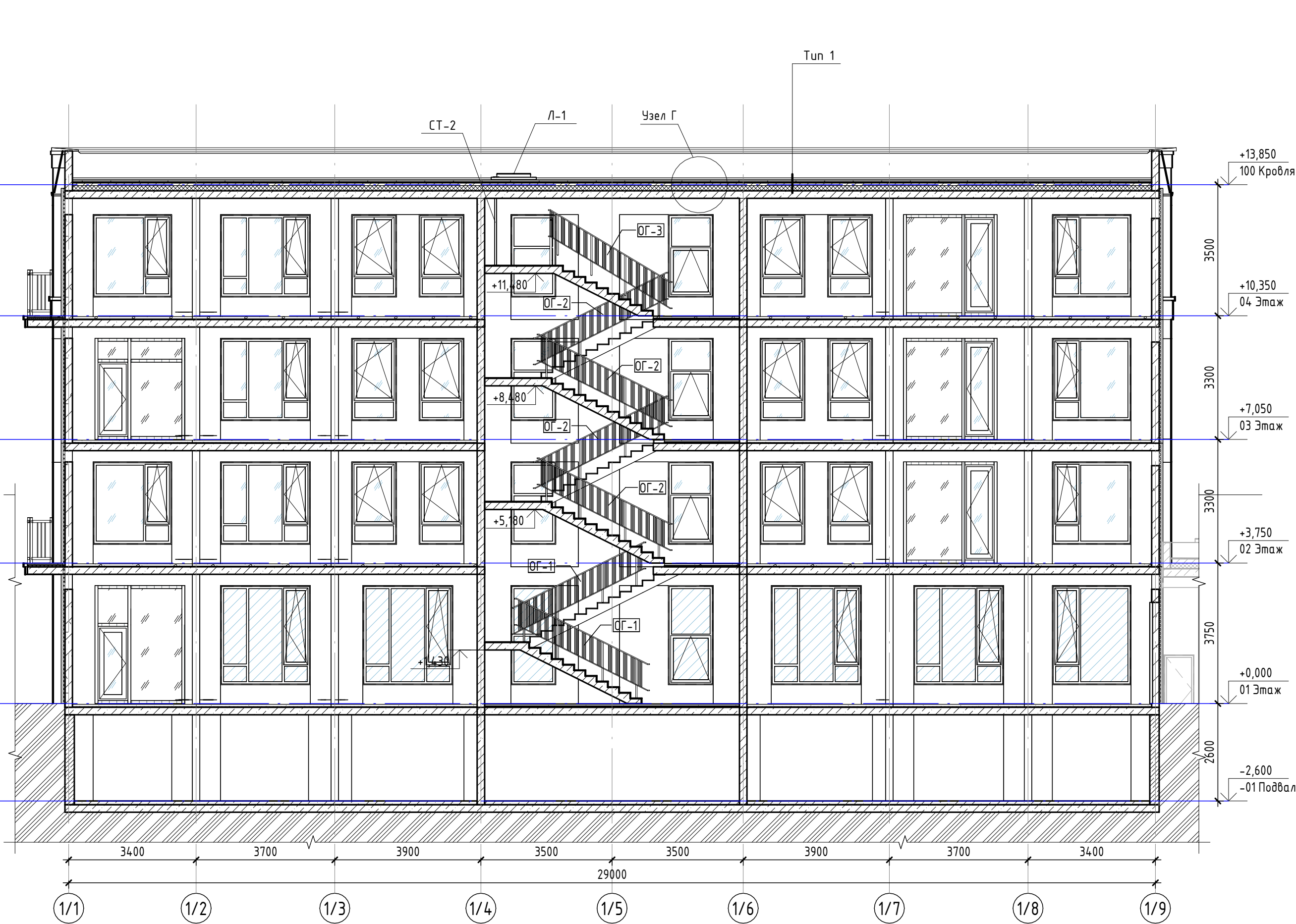
Разрез 2 - 2 ( 1 : 100)
