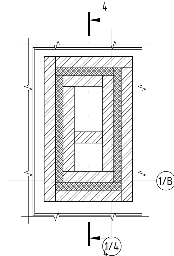
Разрез 4 - 4 ( 1 : 25)
