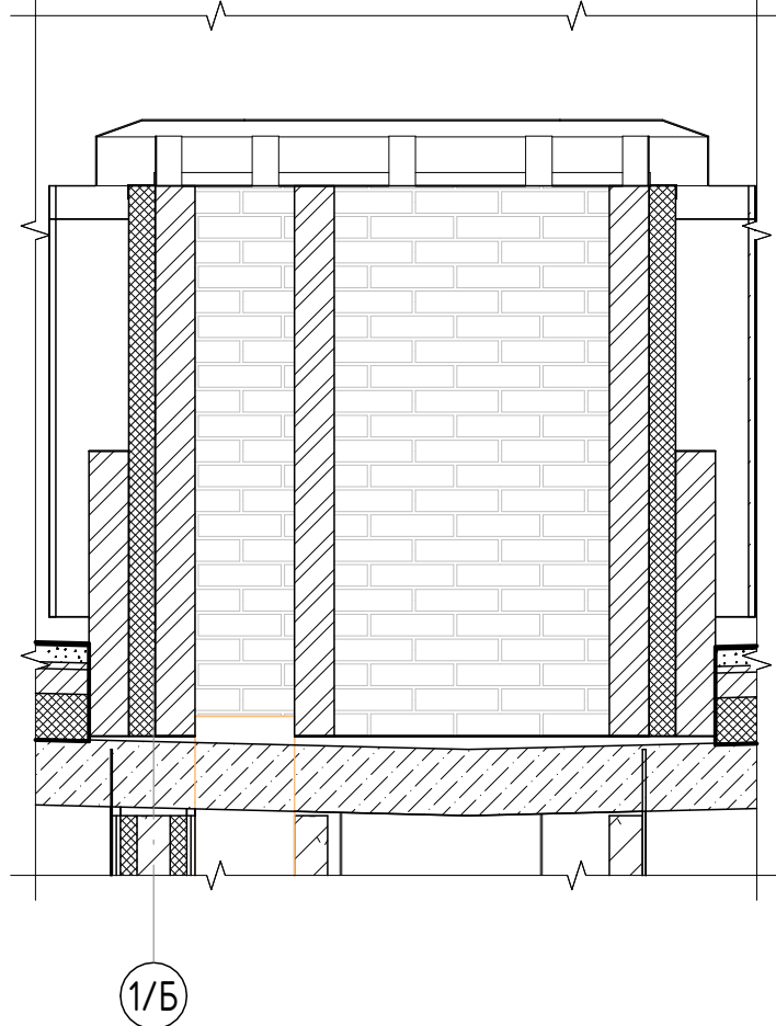
ВШ-7 ( 1 : 25)
