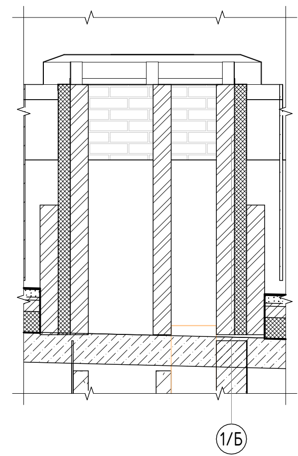
ВШ-6 ( 1 : 25)
