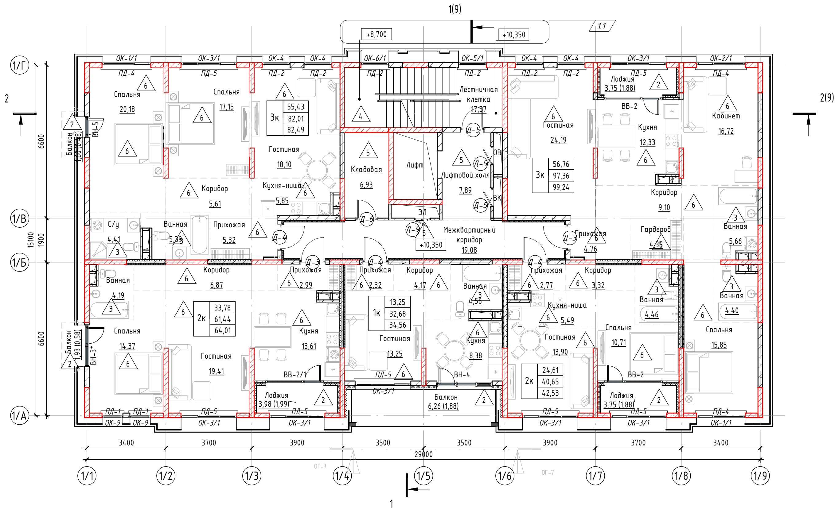
План 4го этажа ( 1 : 100)
