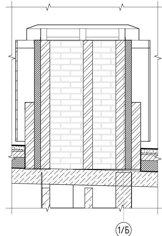
Разрез 7 - 7 ( 1 : 25)
