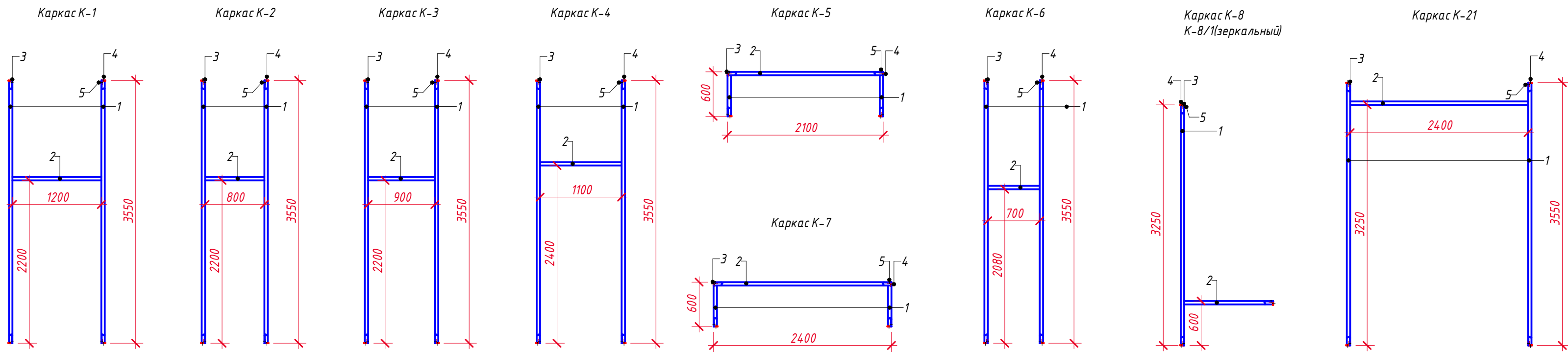
Схемы усиления 1-го этажа
