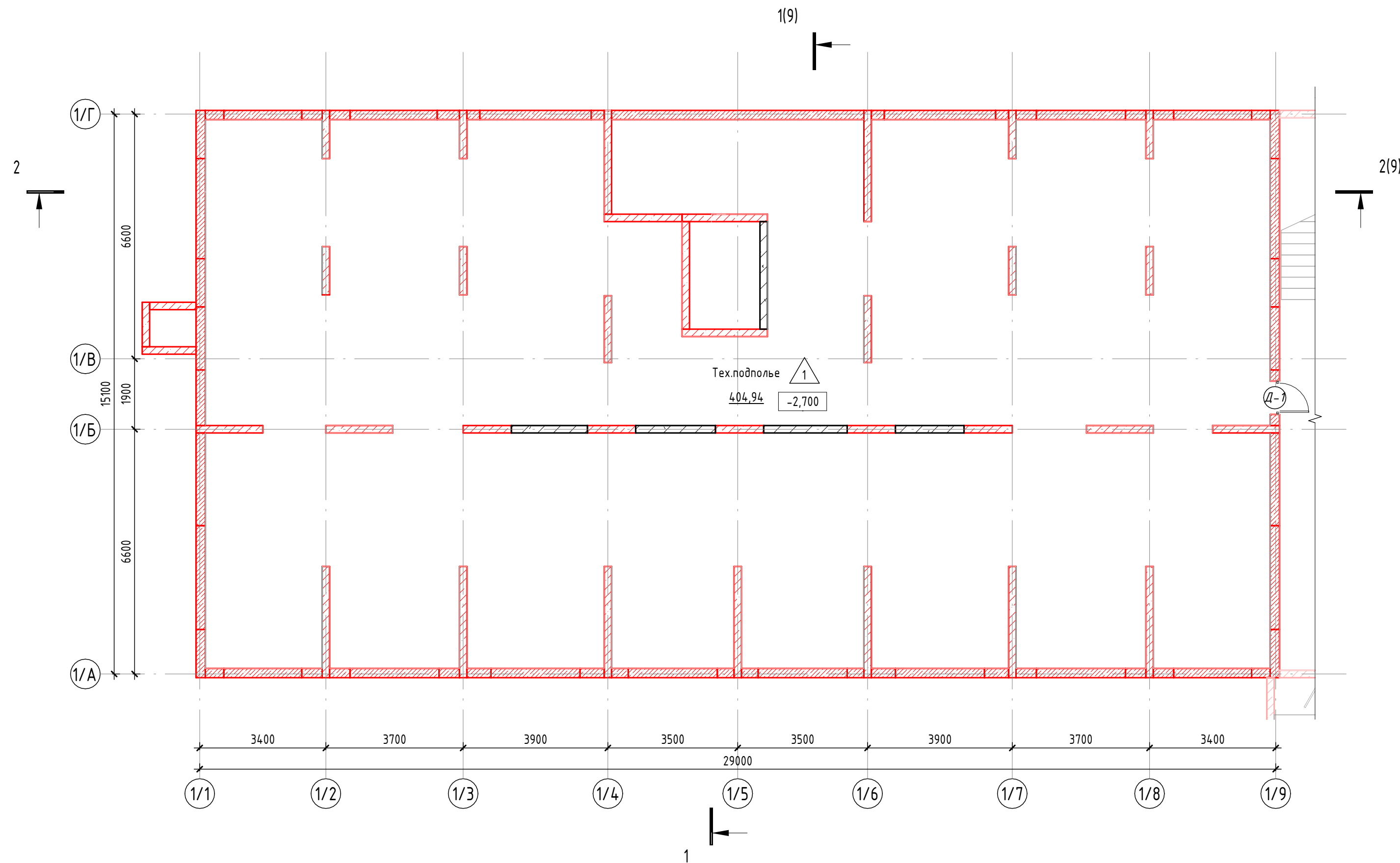
План подвала ( 1 : 100 )
