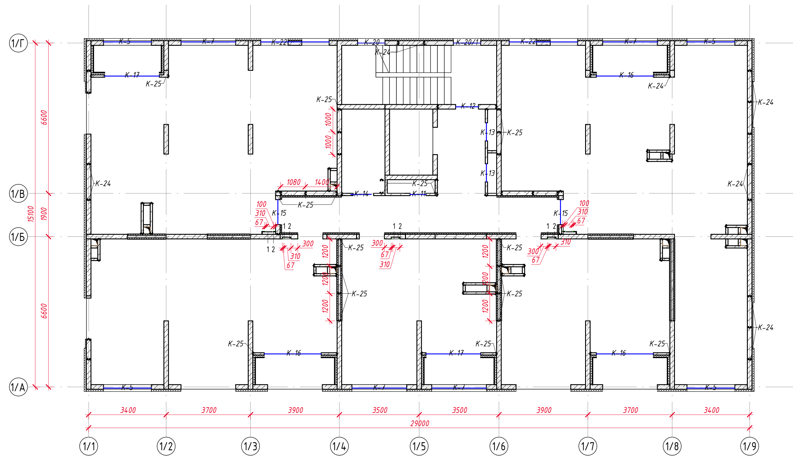
План отверстий и усиления проема 3-го этажа на отм. +7.050 ( 1 : 100)
