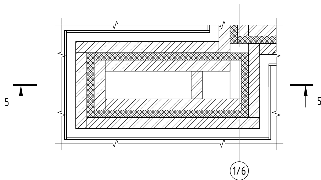
ВШ-5 ( 1 : 25)
