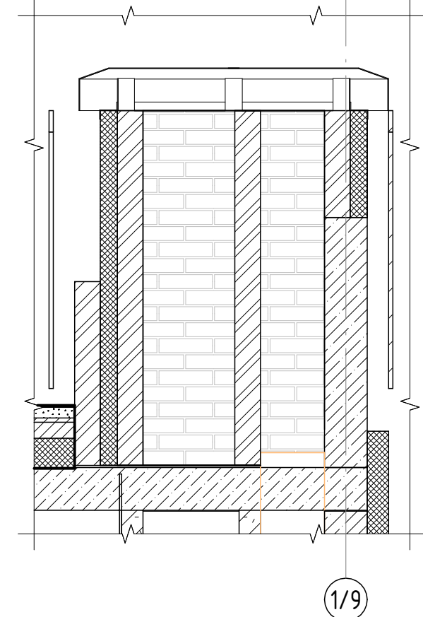
Разрез 9 - 9 ( 1 : 25)
