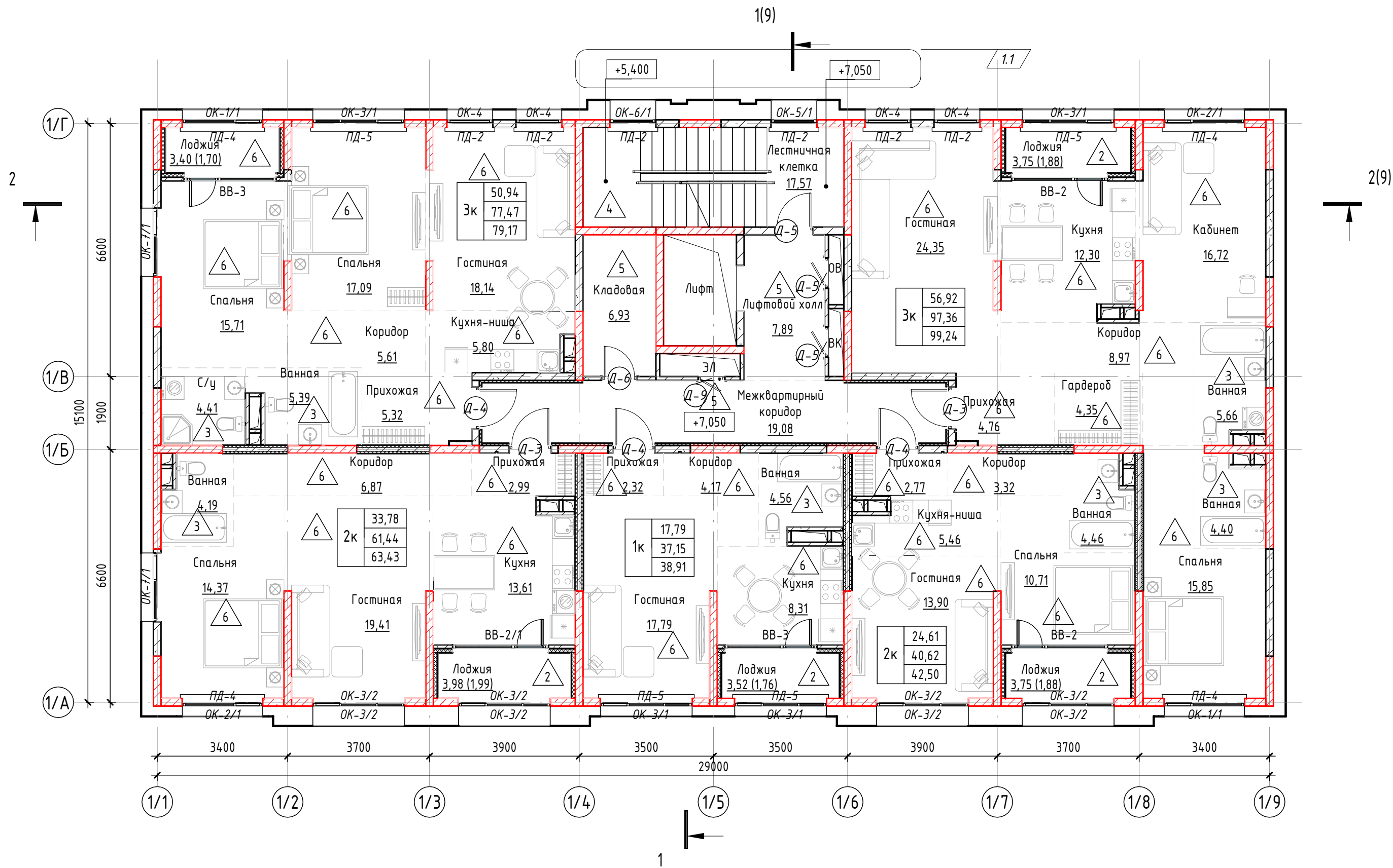
План 3го этажа ( 1 : 100)
