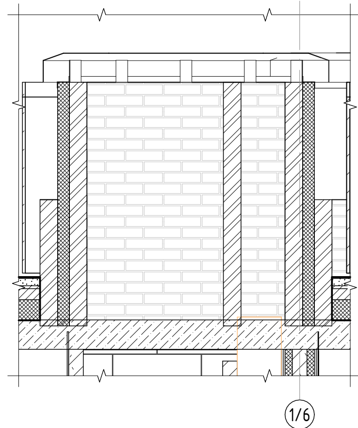
Узел примыкания вентшахт ( 1 : 20)
