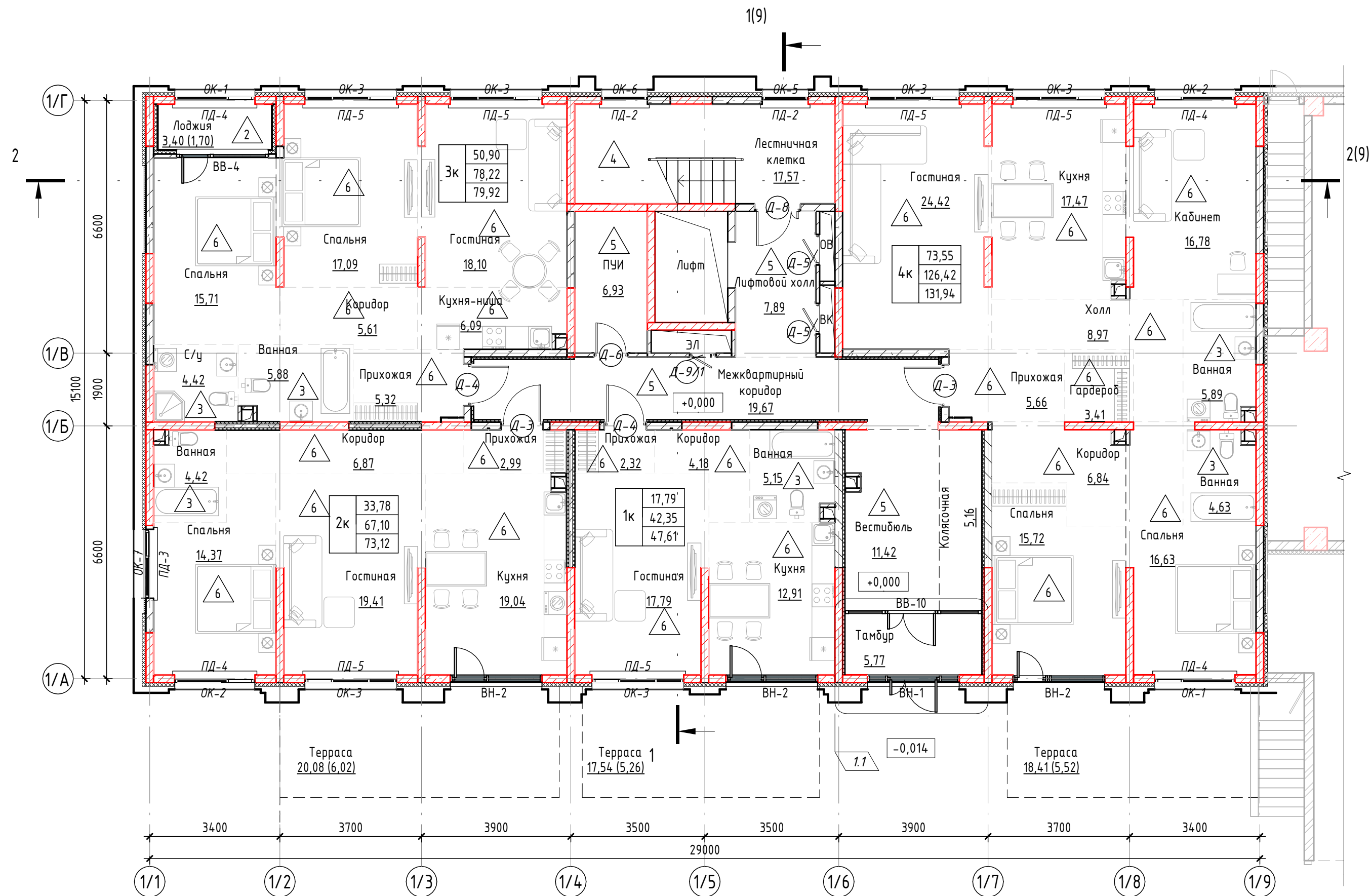
План 1го этажа ( 1 : 100)
