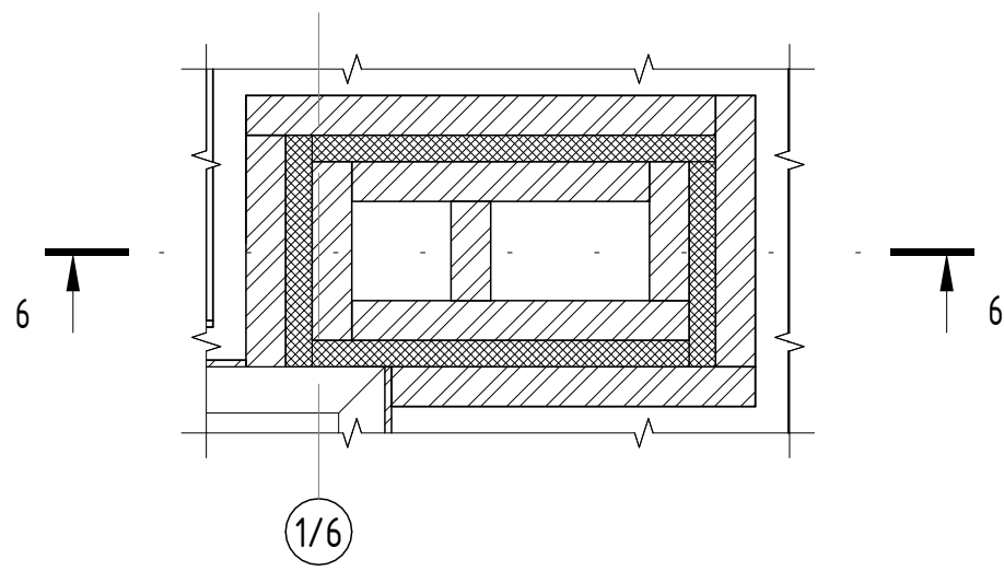
ВШ-6 ( 1 : 25)
