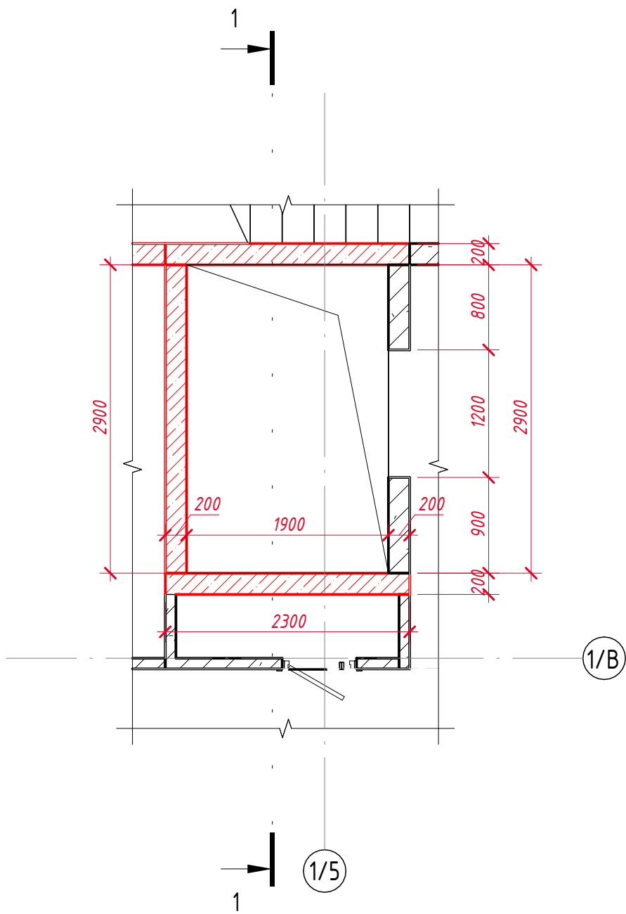
Фрагмент плана лифта ( 1 : 50)
