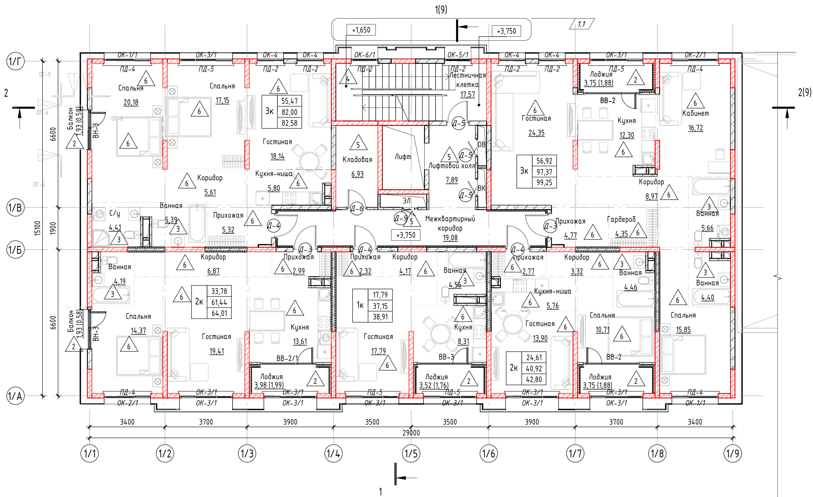
План 2го этажа ( 1 : 100)
