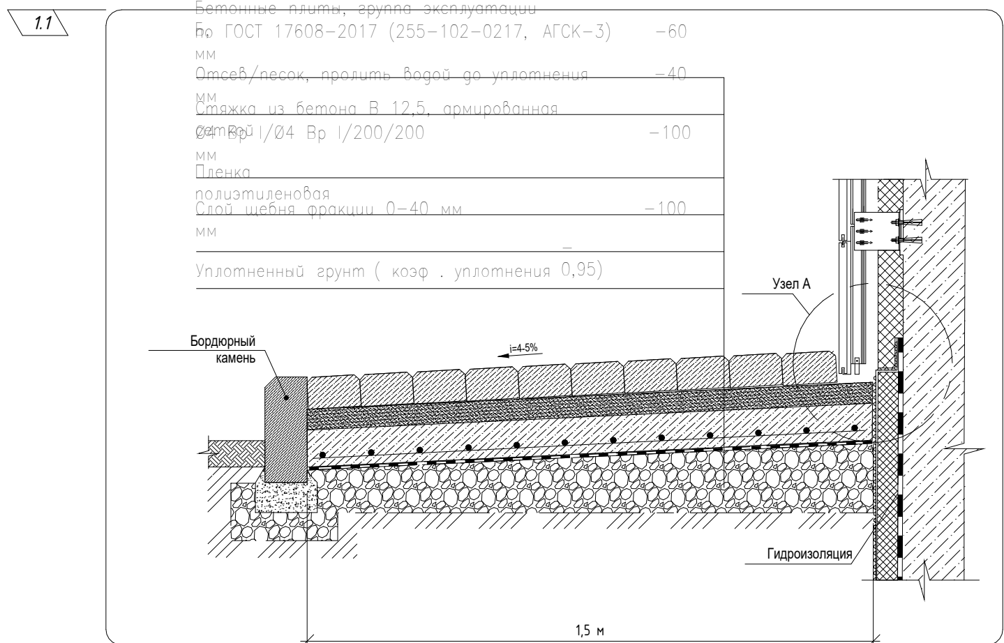
Узел 1
