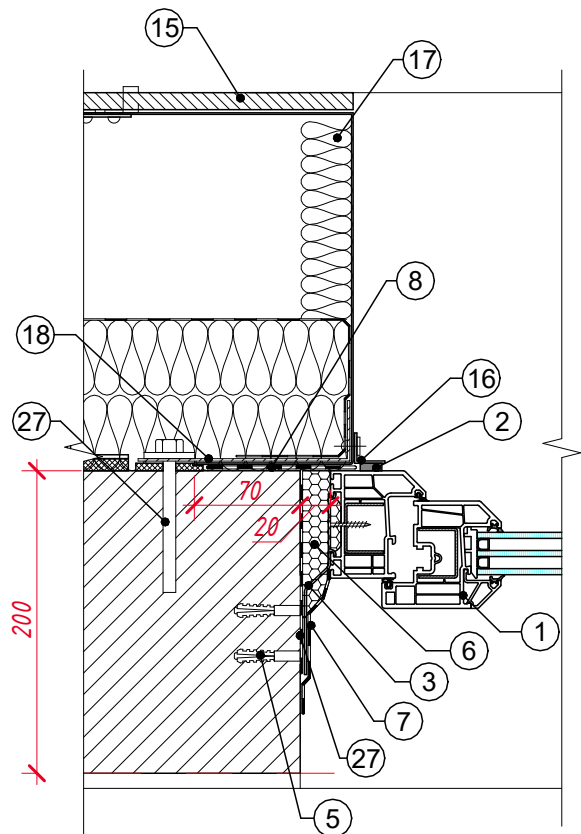
Узел бокового примыкания оконного блока к проему
