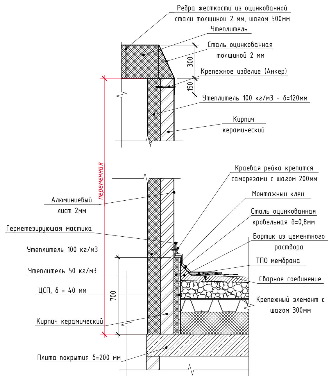
Узел примыкания вентшахт ( 1 : 20)
