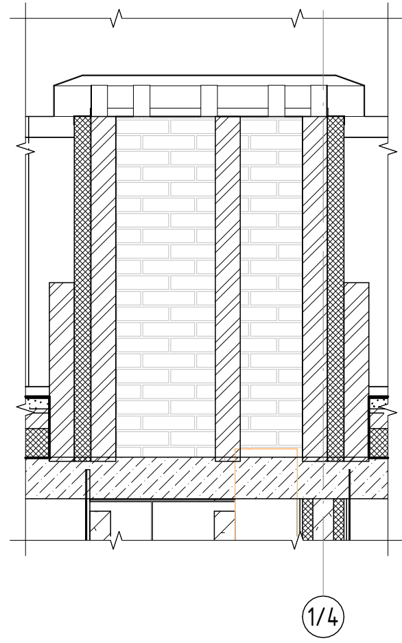
ВШ-8 ( 1 : 25)
