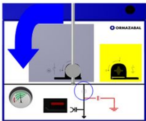
Conectado (Apertura Interruptor)
