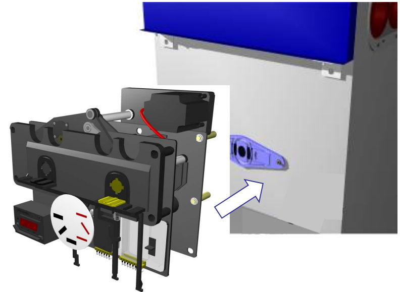
Mecanismo de Maniobra BM
