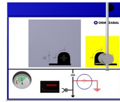
Puesto a Tierra
