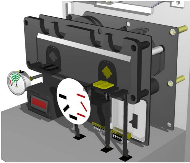
Mecanismo de Maniobra B
