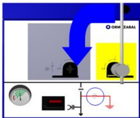
Puesto a Tierra (Apertura Seccionador de PaT)
