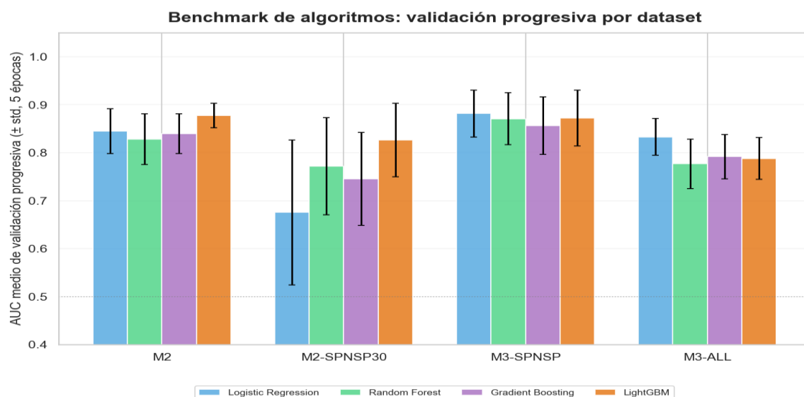
Figura 7.14. AUC medio de validación progresiva ( \pm desviación típica) por algoritmo y conjunto de datos, comparando LightGBM con regresión logística, random forest y gradient boosting genérico. LightGBM es el algoritmo que más veces gana por época individual, aunque la regresión logística lo supere de media en dos de los cuatro conjuntos de datos (7.2.4).
