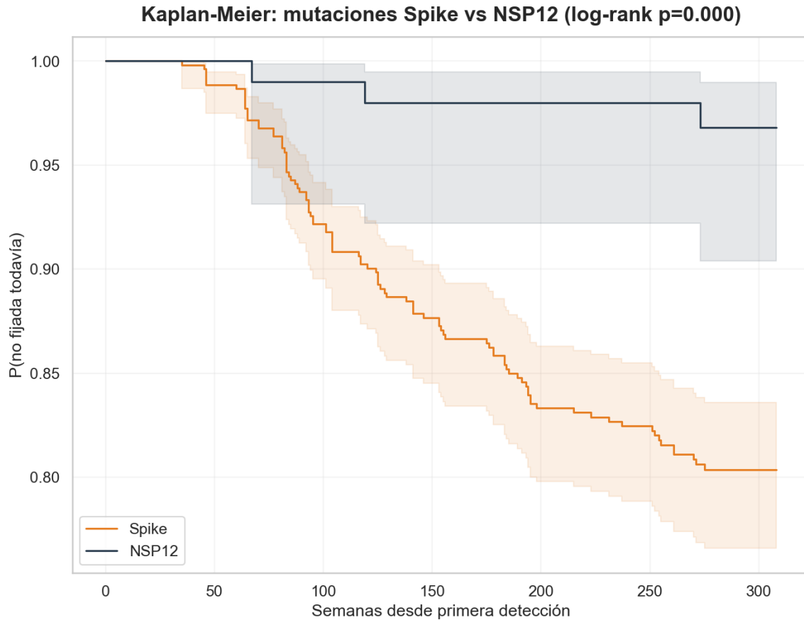
Figura 7.8d. Kaplan-Meier: probabilidad de que una mutación no haya alcanzado aún el umbral de fijación, comparando mutaciones de Spike frente a NSP12.
