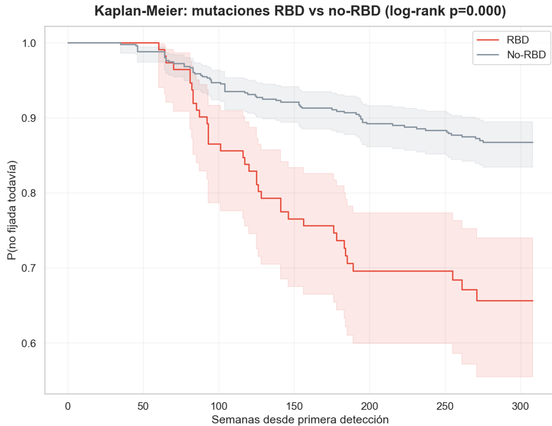
Figura 7.8c. Kaplan-Meier: probabilidad de que una mutación no haya alcanzado aún el umbral de fijación, comparando mutaciones del RBD de Spike frente al resto. Una separación clara entre curvas indica que esa variable adelanta el tiempo hasta la dominancia.
