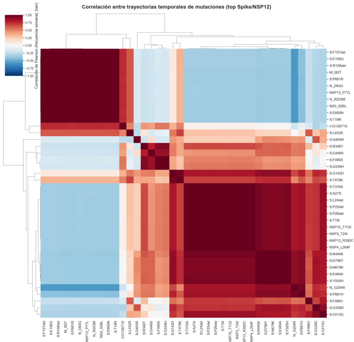
Figura 7.2. Clustermap (matriz de correlación con las mutaciones reordenadas por similitud) de la correlación de Pearson entre las trayectorias temporales de frecuencia de las mutaciones top de Spike/NSP12. Los bloques de color intenso agrupan mutaciones cuya frecuencia sube y baja de forma sincronizada, candidatas a convergencia evolutiva o a pertenecer a la misma familia genómica.
