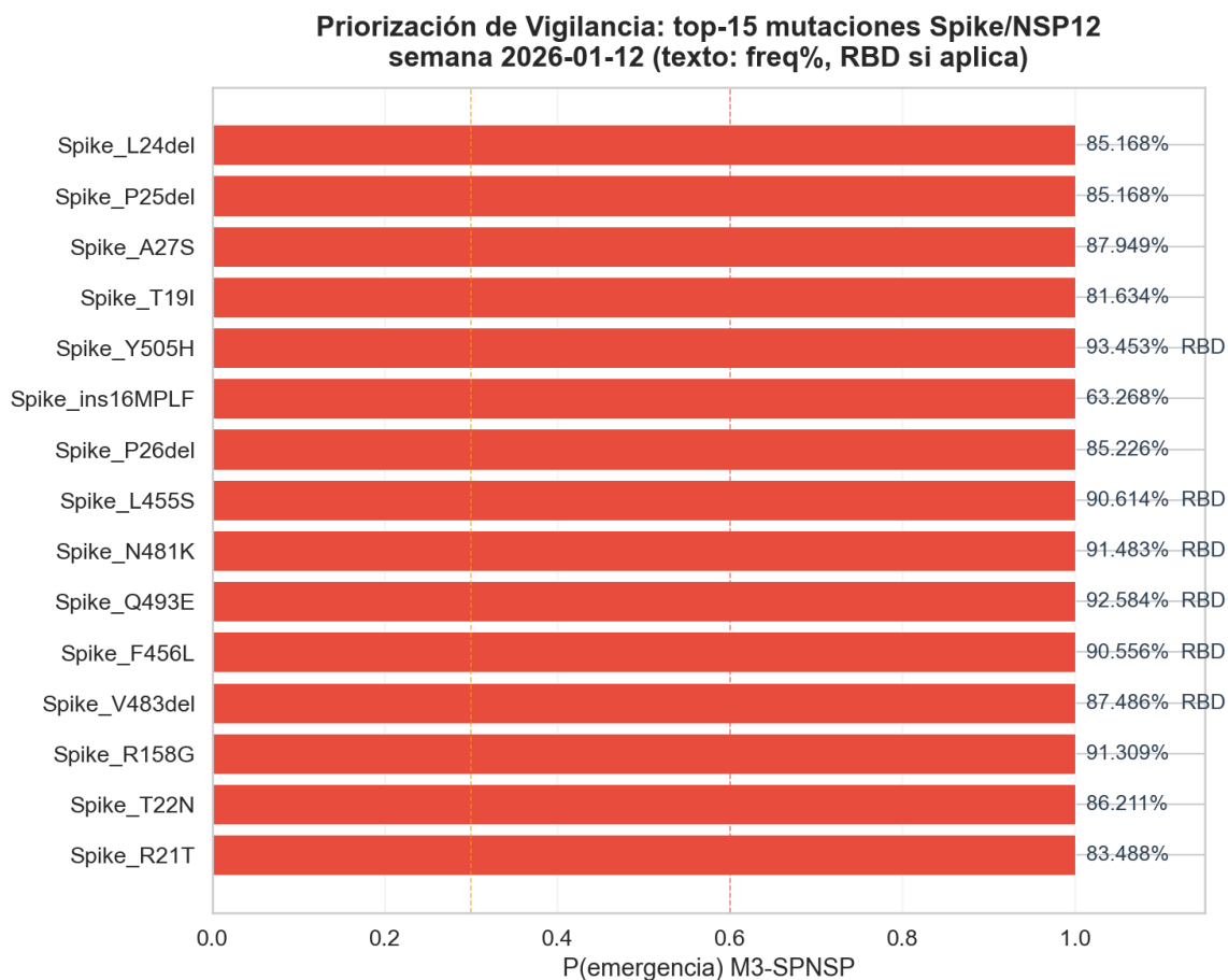
Figura 7.10c. Priorización de vigilancia activa: top-15 mutaciones Spike/NSP12 por probabilidad calibrada de emergencia (clasificador M3-SPNSP), marcando las que pertenecen al RBD. Las familias y mutaciones por encima del umbral HIGH son las prioritarias para vigilancia reforzada.
