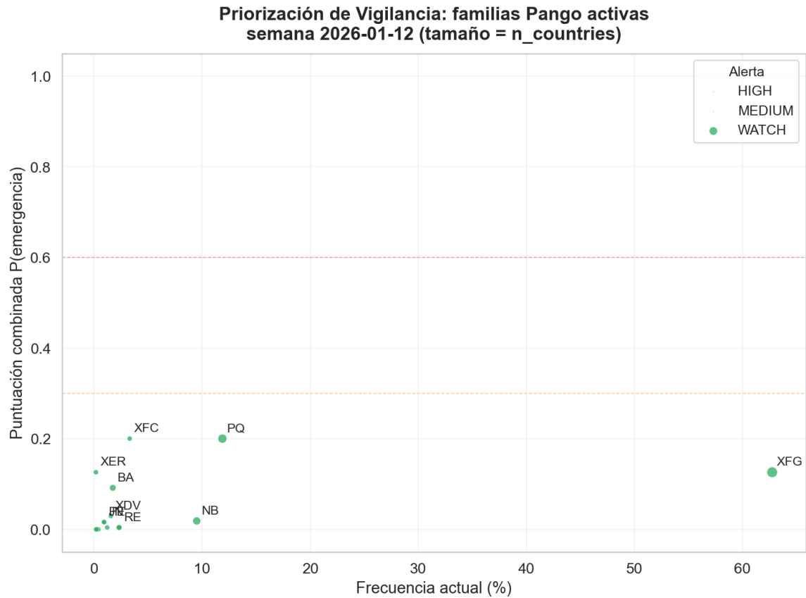
Figura 7.10a. Priorización de vigilancia activa: cada burbuja es una familia Pango, su tamaño representa el número de países donde se ha detectado y su posición vertical la probabilidad calibrada de alcanzar el umbral de dominancia.
