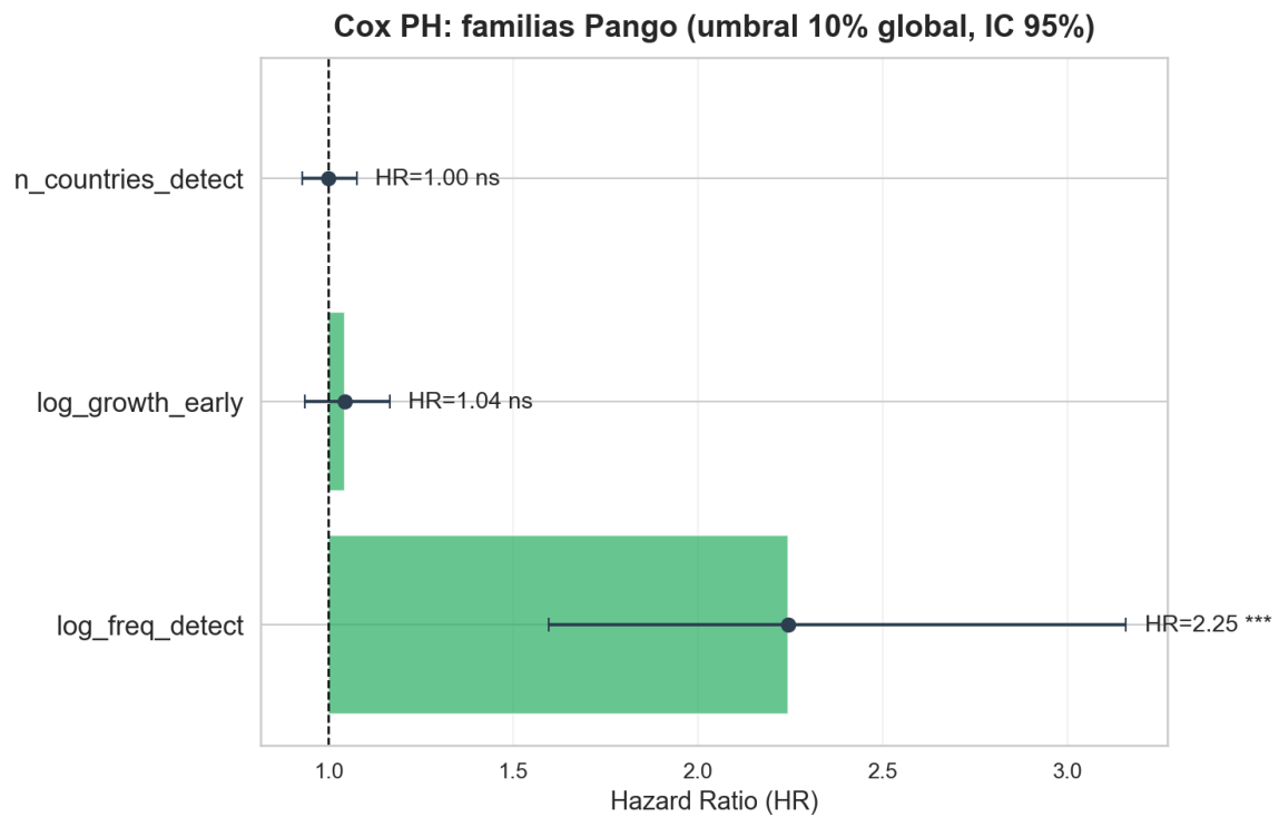
Figura 7.9a. Hazard ratios con intervalo de confianza del 95% del modelo Cox PH para familias Pango (umbral de dominancia 10% global): un HR mayor que 1 indica que valores altos de esa variable aceleran la dominancia, y un intervalo que no cruza el valor 1 indica significación estadística.
