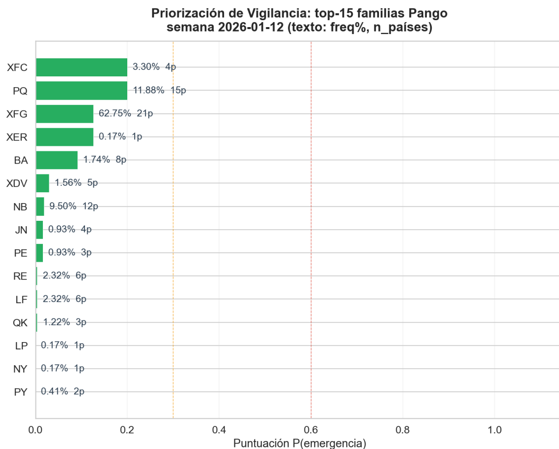
Figura 7.10b. Priorización de vigilancia activa: top-15 familias Pango por probabilidad calibrada de emergencia, con su frecuencia actual y número de países.
