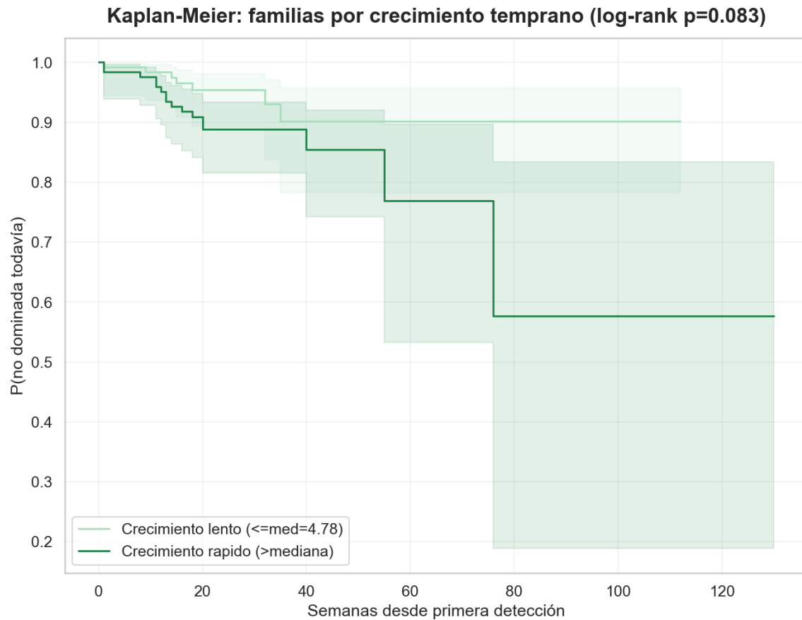
Figura 7.8b. Kaplan-Meier: probabilidad de que una familia no haya alcanzado aún el umbral de dominancia, según su velocidad de crecimiento temprano (lento vs. rápido).
