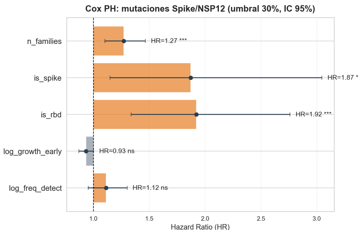
Figura 7.9b. Hazard ratios con intervalo de confianza del 95% del modelo Cox PH para mutaciones Spike/NSP12 (umbral de fijación 30%). la pertenencia al RBD, a Spike y la convergencia evolutiva histórica son los predictores más fuertes y significativos ( p < 0.05 ); la frecuencia en el momento de detección no lo es a este nivel de mutación individual ( p = 0.167 , Tabla 7.5).
