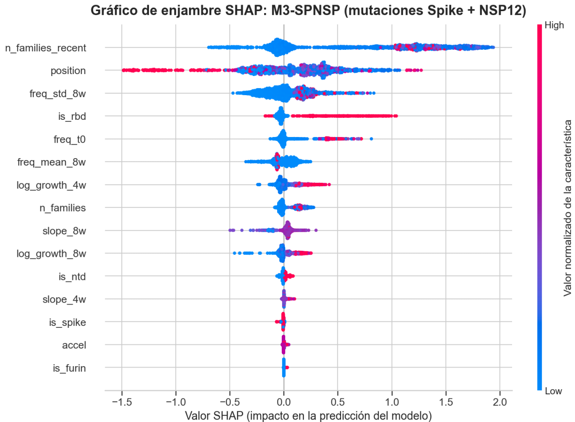
Figura 8.6. Gráfico de enjambre (beeswarm) de valores SHAP para M3-SPNSP: cada punto es una observación (mutación, semana), su posición horizontal indica si esa característica empujó la predicción hacia una mayor o menor probabilidad de dominancia, y el color indica si el valor de la característica en esa observación fue alto (rojo) o bajo (azul).
