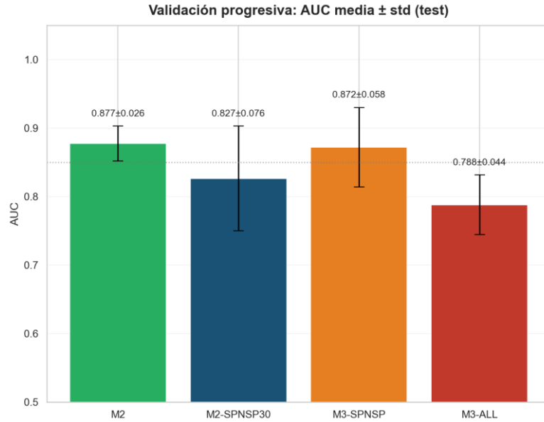
Figura 8.3b. AUC media \pm desviación típica de la validación progresiva (test), por conjunto de datos. Es consistentemente igual o inferior al AUC de la partición temporal fija, la firma esperada cuando no hay fuga de información entre entrenamiento y validación.
