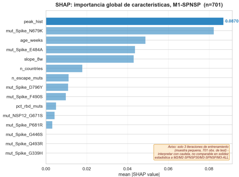
Figura 8.5g. Importancia SHAP media ( |SHAP| ) en M1-SPNSP (M1 + mutaciones Spike/NSP12). Misma salvedad: solo 3 iteraciones de entrenamiento, la muestra más pequeña de las siete.
