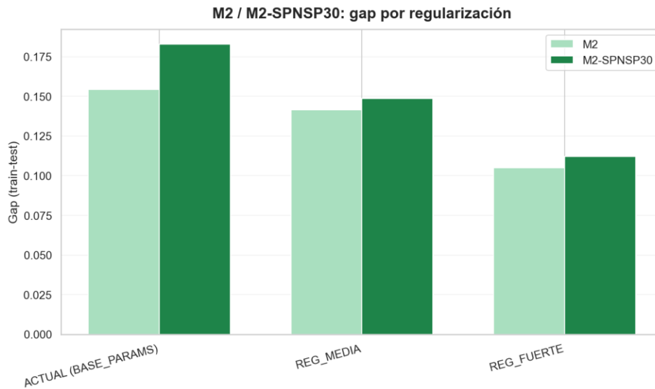
Figura 8.4b. Sensibilidad de M2 y M2-SPNSP30 a la fuerza de regularización de LightGBM: diferencia train-test (gap de sobreajuste) para las mismas configuraciones. La configuración final, más regularizada, mejora el AUC de test y reduce el gap a la vez respecto a la configuración base, un resultado poco intuitivo que solo se confirmó probándolo.
