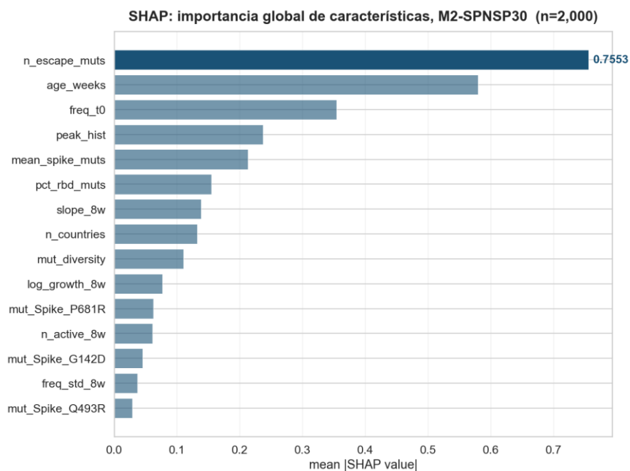
Figura 8.5b. Importancia SHAP media ( |SHAP| ) en M2-SPNSP30 (familias Pango + 30 mutaciones Spike/NSP12 más informativas).
