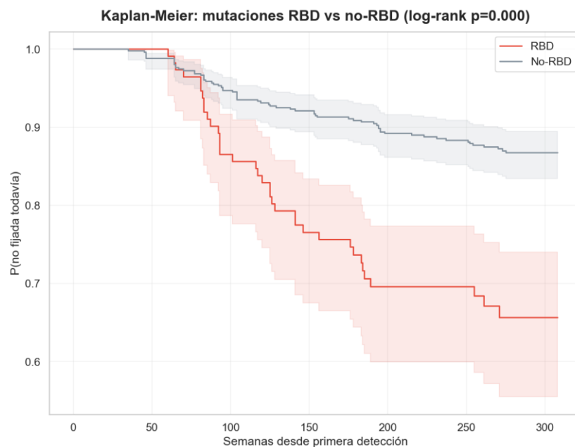
Figura 9.1c. Kaplan-Meier: probabilidad de que una mutación no haya alcanzado aún el umbral de fijación, comparando mutaciones del RBD de Spike frente al resto. Una separación clara entre curvas indica que esa variable adelanta el tiempo hasta la dominancia.
