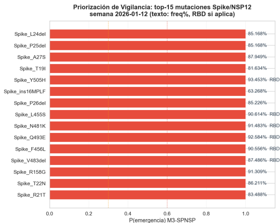
Figura 10.1c. Priorización de vigilancia activa: top-15 mutaciones Spike/NSP12 por probabilidad calibrada de emergencia (clasificador M3-SPNSP), marcando las que pertenecen al RBD. Las familias y mutaciones por encima del umbral HIGH son las prioritarias para vigilancia reforzada.
