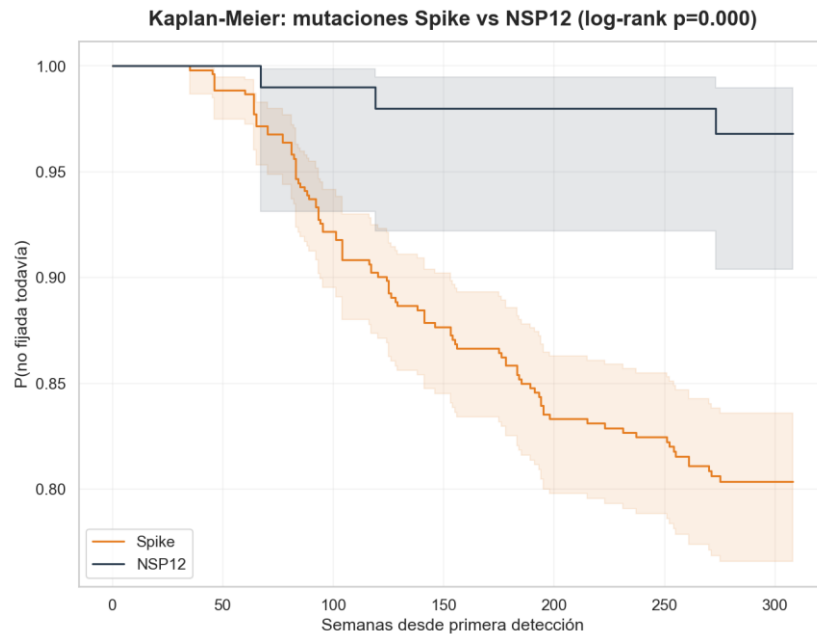
Figura 9.1d. Kaplan-Meier: probabilidad de que una mutación no haya alcanzado aún el umbral de fijación, comparando mutaciones de Spike frente a NSP12.
