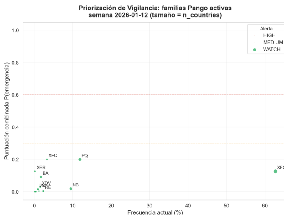
Figura 10.1a. Priorización de vigilancia activa: cada burbuja es una familia Pango, su tamaño representa el número de países donde se ha detectado y su posición vertical la probabilidad calibrada de alcanzar el umbral de dominancia.
