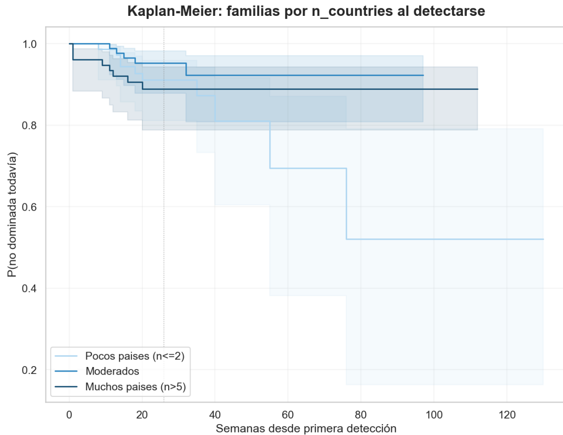
Figura 9.1a. Kaplan-Meier: probabilidad de que una familia no haya alcanzado aún el umbral de dominancia, según el número de países en que se detectó tempranamente.
