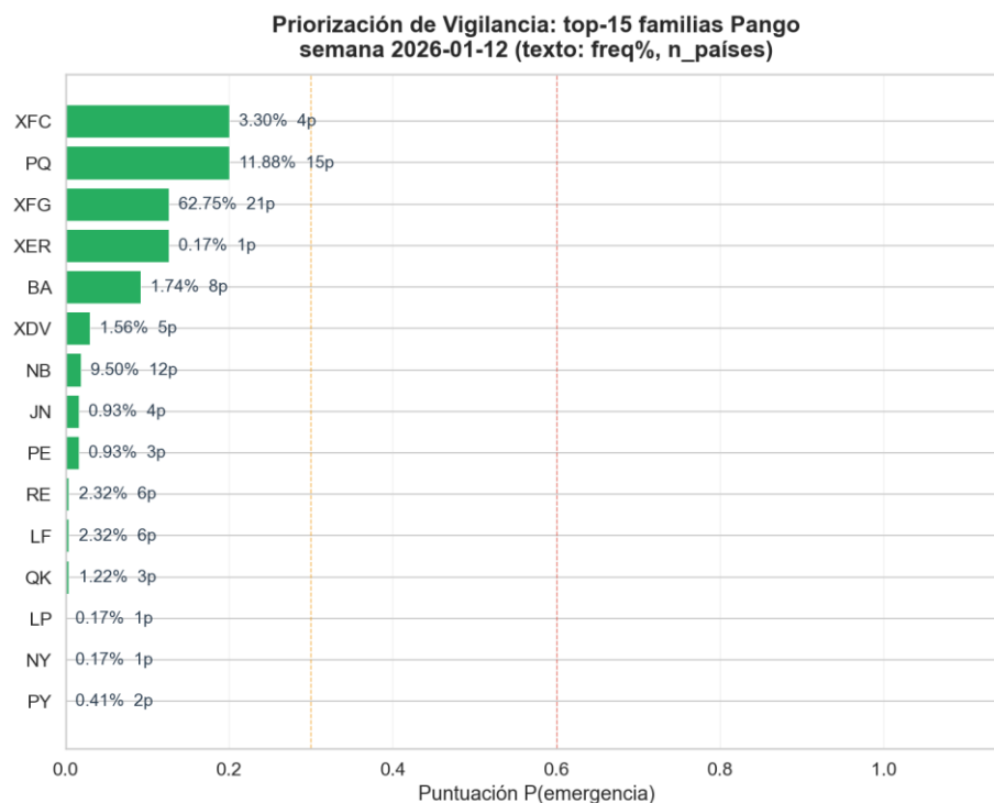
Figura 10.1b. Priorización de vigilancia activa: top-15 familias Pango por probabilidad calibrada de emergencia, con su frecuencia actual y número de países.
