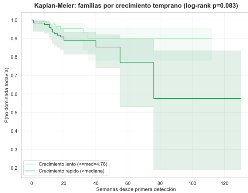
Figura 9.1b. Kaplan-Meier: probabilidad de que una familia no haya alcanzado aún el umbral de dominancia, según su velocidad de crecimiento temprano (lento vs. rápido).
