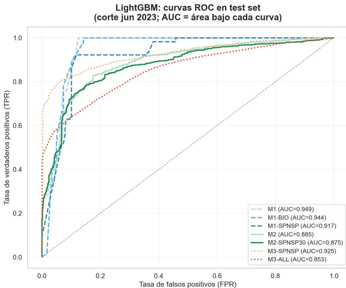
Figura 8.2a. Curvas ROC de los siete conjuntos de datos en test (corte junio 2023): el área bajo cada curva es el AUC de test.
