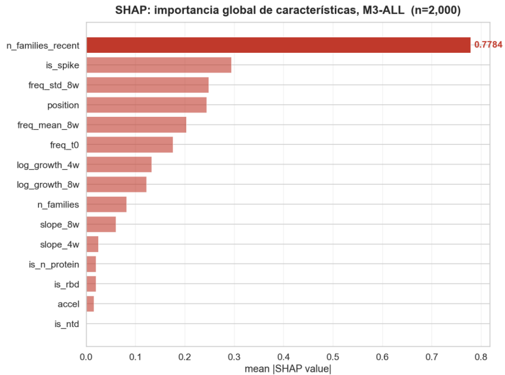
Figura 8.5d. Importancia SHAP media ( |SHAP| ) en M3-ALL (todas las mutaciones del genoma con señal real). La característica dominante cambia con la granularidad: la frecuencia histórica en M1, el escape inmune en M2 y la convergencia evolutiva reciente en los modelos de mutación individual (M3).
