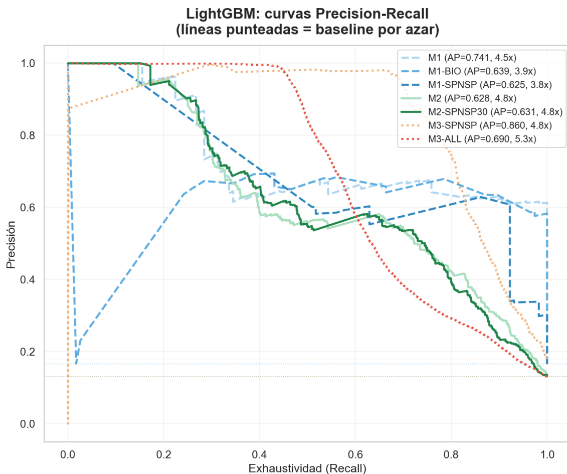
Figura 8.2b. Curvas Precision-Recall de los siete conjuntos de datos en test, con la línea punteada como referencia del baseline por azar de cada uno.
