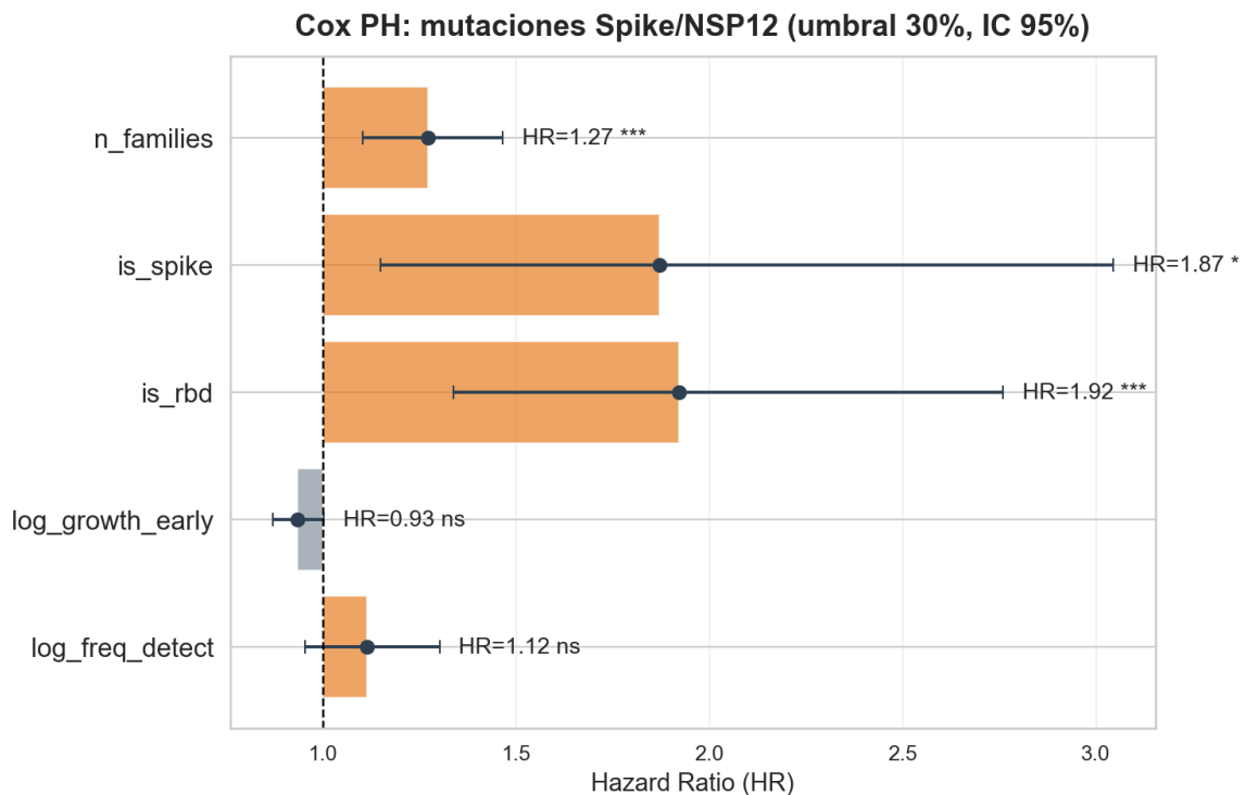
Figura 9.2b. Hazard ratios con intervalo de confianza del 95% del modelo Cox PH para mutaciones Spike/NSP12 (umbral de fijación 30%). La pertenencia al RBD, a Spike y la convergencia evolutiva histórica son los predictores más fuertes y significativos ( p < 0.05 ); la frecuencia en el momento de detección no lo es a este nivel de mutación individual ( p = 0.167 , Tabla 9.3).
