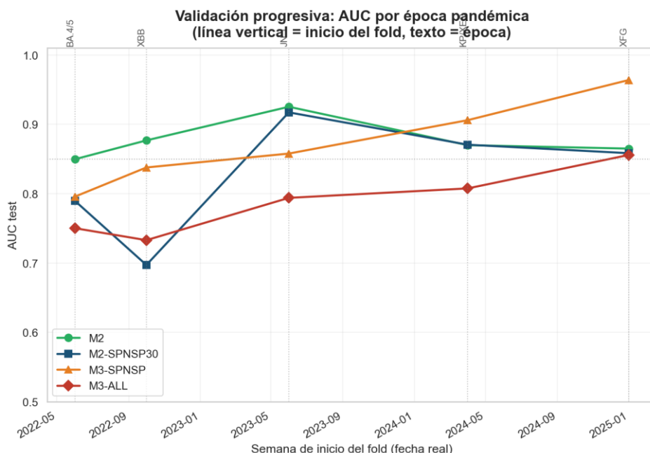
Figura 8.3a. AUC de validación progresiva por época pandémica, en el eje real de fechas de inicio de cada fold, para los cuatro conjuntos de datos evaluados.
