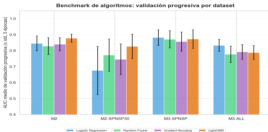
Figura 8.1. AUC medio de validación progresiva ( \pm desviación típica) por algoritmo y conjunto de datos, comparando LightGBM con regresión logística, random forest y gradient boosting genérico. LightGBM es el algoritmo que más veces gana por época individual, aunque la regresión logística lo supere de media en dos de los cuatro conjuntos de datos (8.1).
