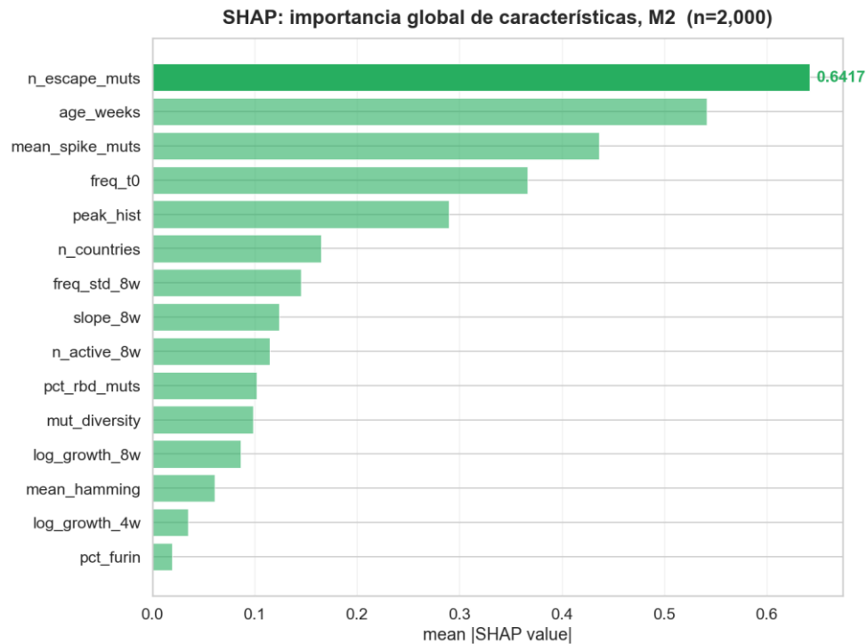
Figura 8.5a. Importancia SHAP media ( |SHAP| ) en M2 (familias Pango, características temporales + biológicas): mide cuánto desplaza cada característica la predicción del modelo respecto a la media.
