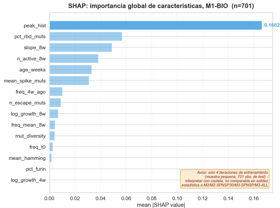
Figura 8.5f. Importancia SHAP media ( |SHAP| ) en M1-BIO (M1 + perfil biológico). Misma salvedad que la Figura 8.5e: solo 4 iteraciones de entrenamiento.
