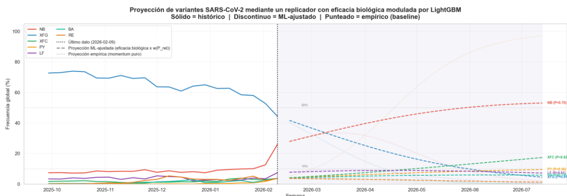
Figura 10.3. Proyección semanal de frecuencia de las variantes activas desde el corte de datos (línea sólida = histórico), comparando el escenario ajustado por LightGBM (línea discontinua) con el modelo de referencia puramente empírico (línea punteada). El modelo de referencia sobreestima el crecimiento de PY hasta un falso dominio futuro, un error que la modulación por LightGBM corrige.
