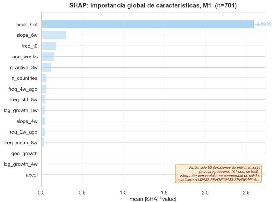
Figura 8.5e. Importancia SHAP media ( |SHAP| ) en M1 (clados Nextclade en fase pre-emergencia). Se incluye con una nota de aviso: entrenado con muy pocas iteraciones (63) frente a los cuatro conjuntos de datos principales, por lo que su importancia SHAP debe interpretarse con cautela.
