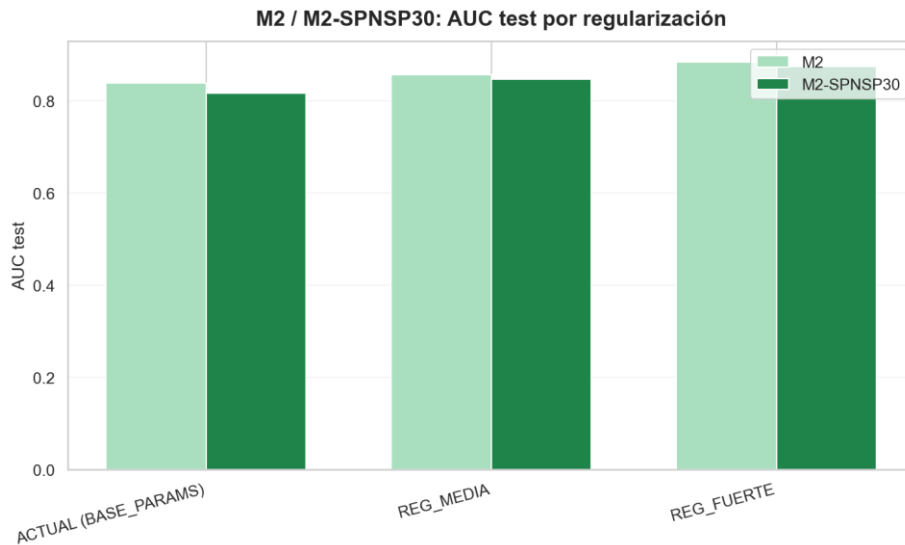
Figura 8.4a. Sensibilidad de M2 y M2-SPNSP30 a la fuerza de regularización de LightGBM: AUC de test para distintas configuraciones de hiperparámetros.
