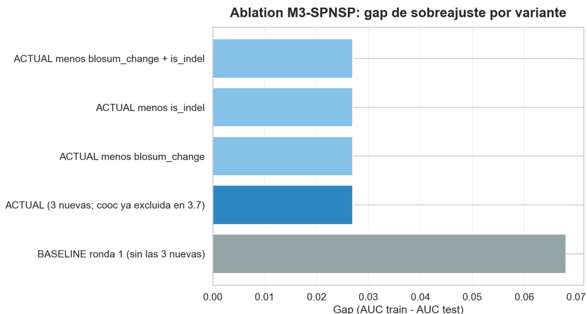
Figura 6.1b. Ablation de M3-SPNSP: diferencia train-test o gap de sobreajuste al quitar las mismas características candidatas. Juntas reducen el gap a la mitad, la razón por la que se excluyeron del modelo final.
