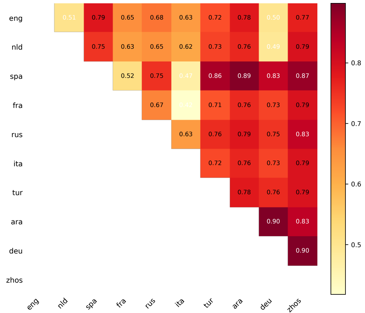
Typological distance (average)
