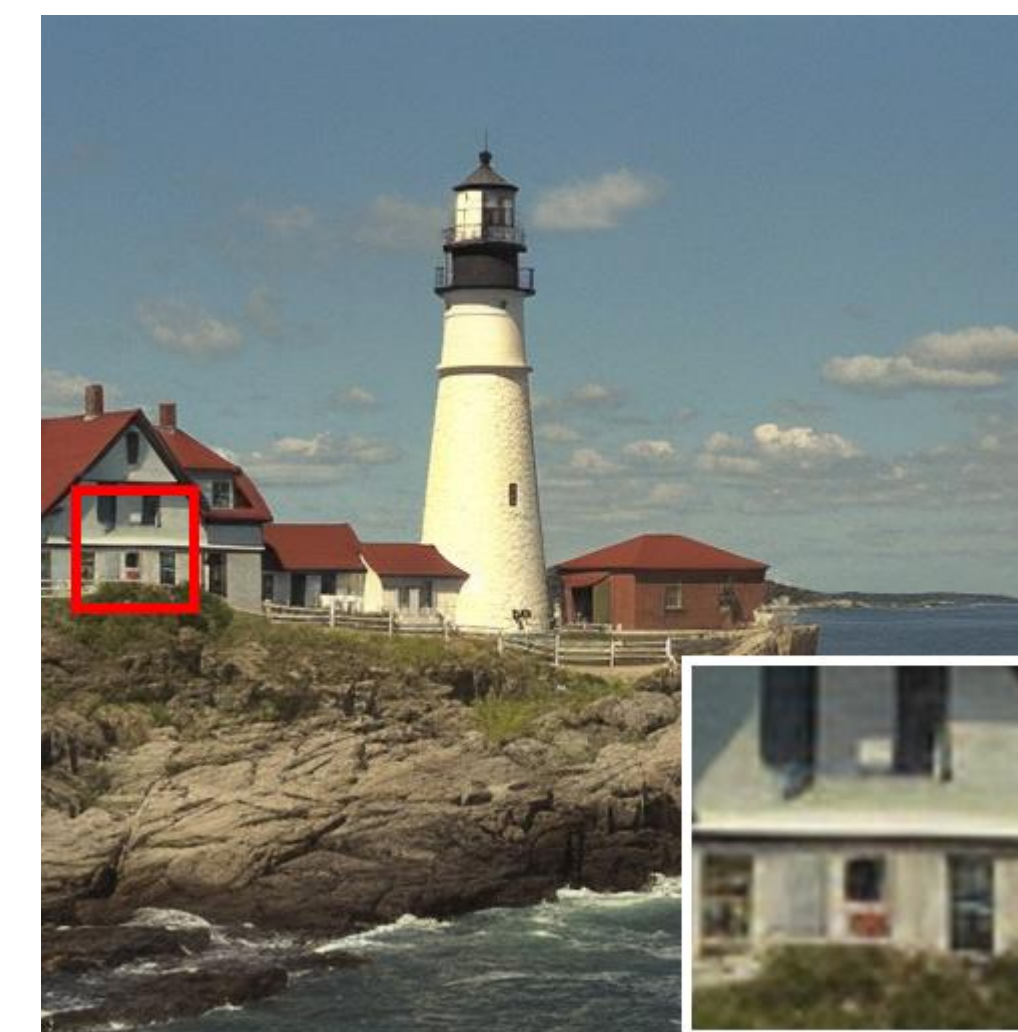
RDEIC
