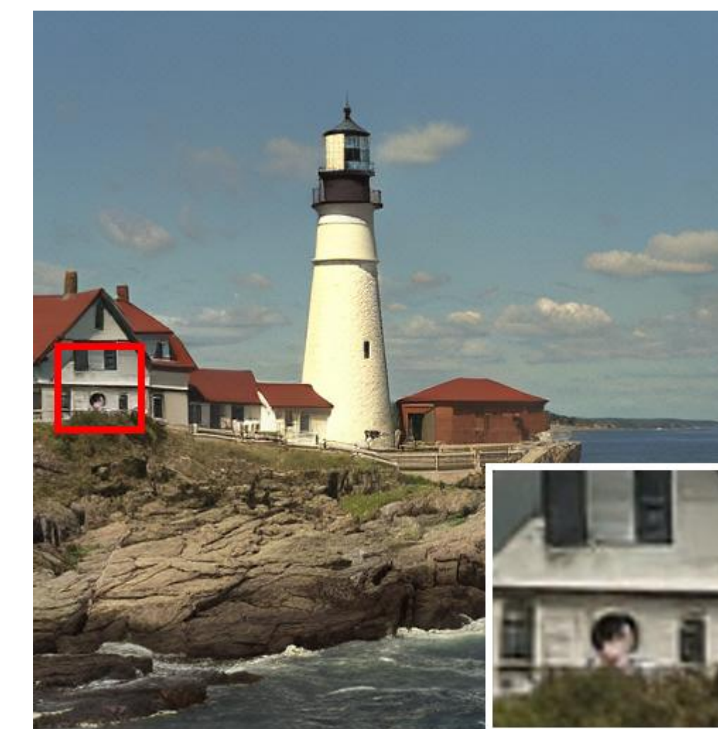
EF-LIC (Ours)
