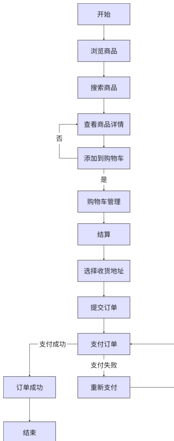
图 4-3 商品购买流程图
