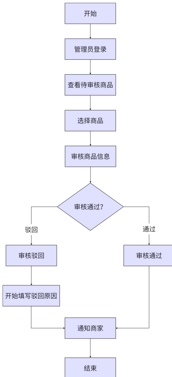
图 4-4 商品审核流程图
