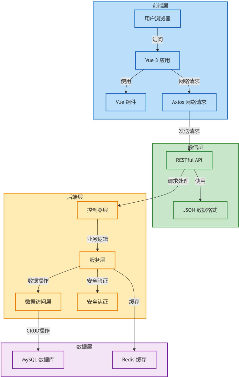
图 4- 1 架构设计图
