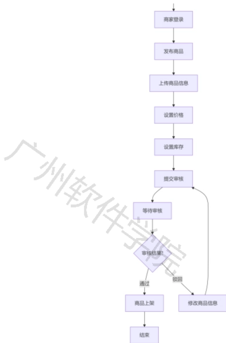
图4- 2 商品发布流程活动图
