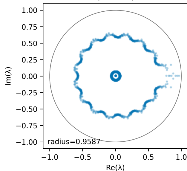
(d) Companion spectrum
