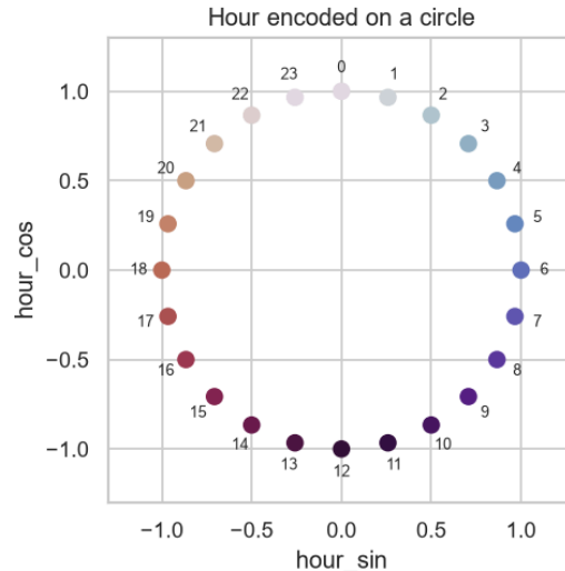
รูปที่ 5.1 ชั่วโมงหลังแปลงเป็น (hour_sin, hour_cos) เรียงเป็นวงกลม
