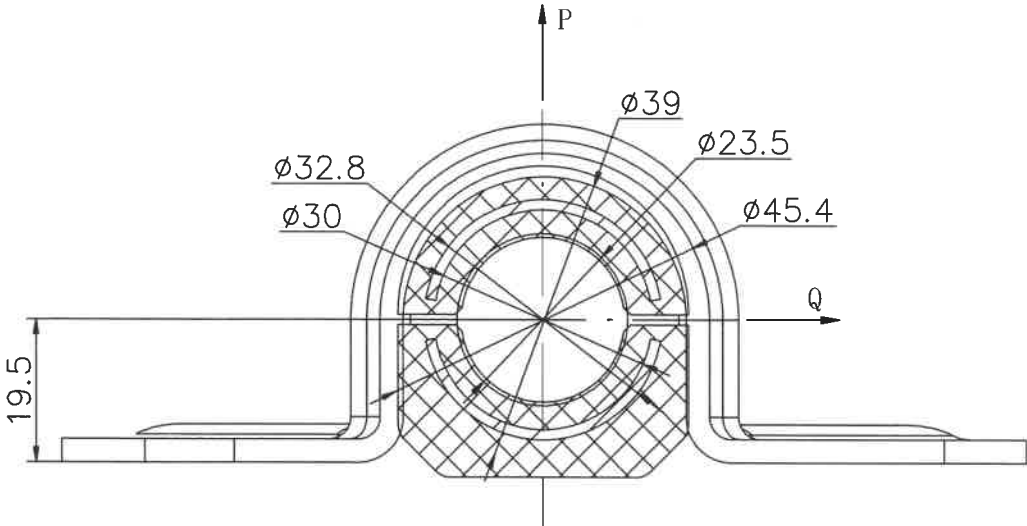
衬套安装状态示意图
