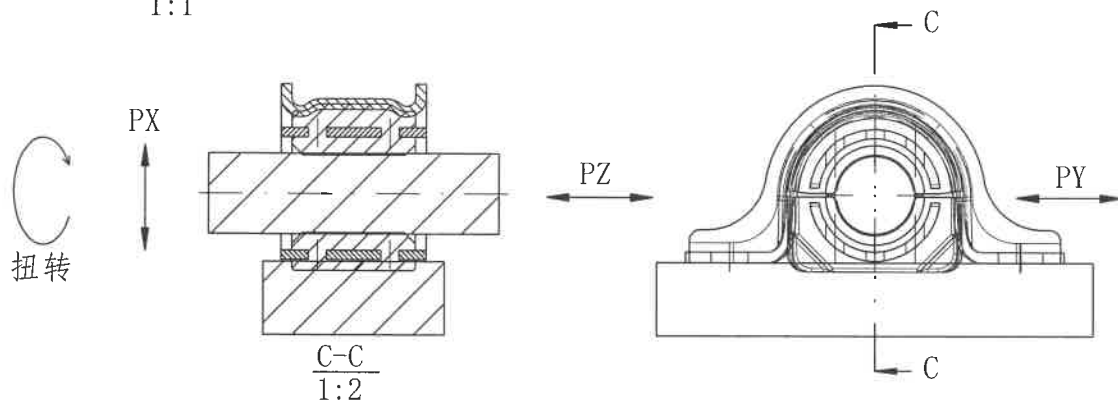
图1. 稳定杆衬套刚度试验装夹示意图
