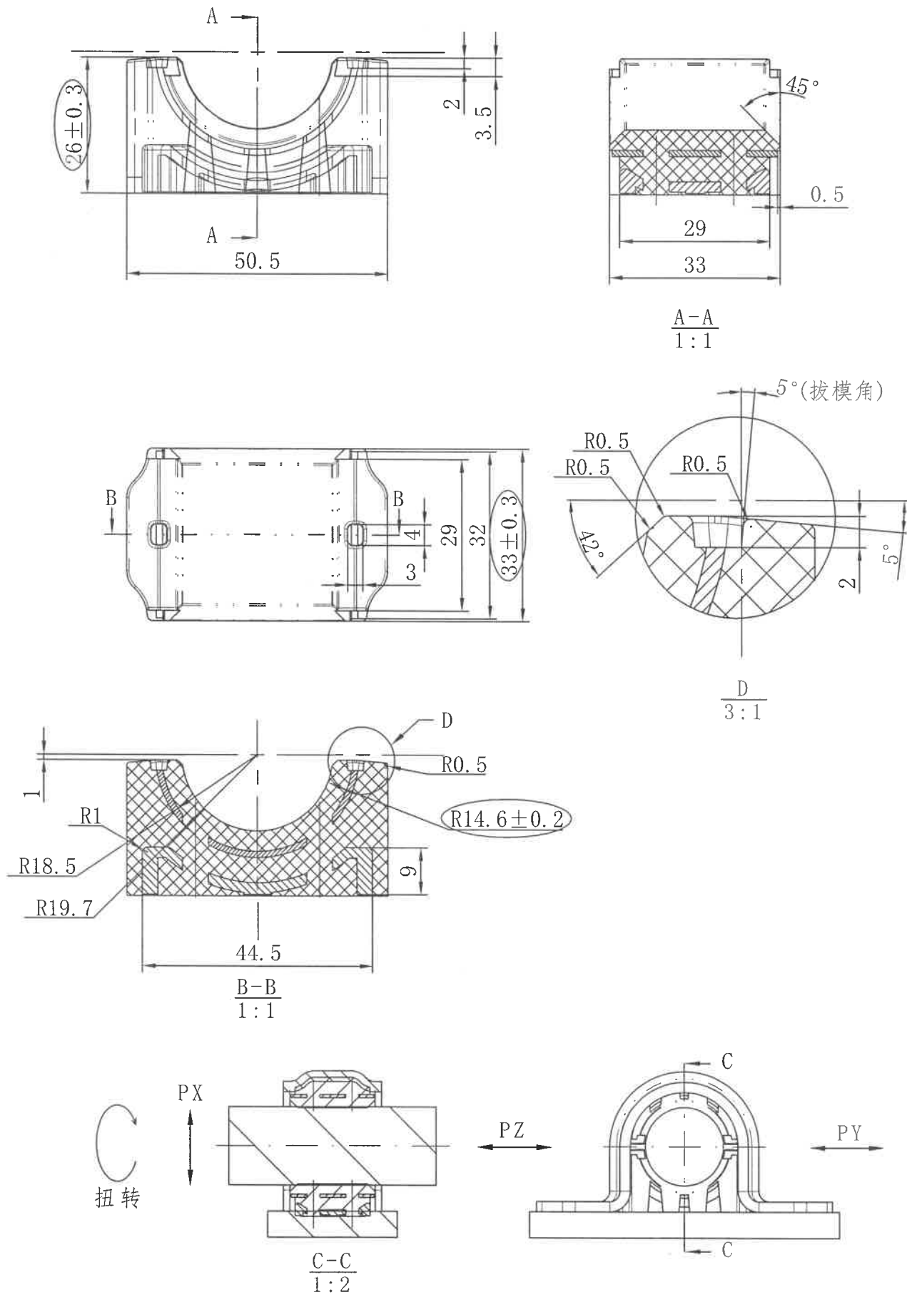
图1. 稳定杆衬套刚度试验装夹示意图
