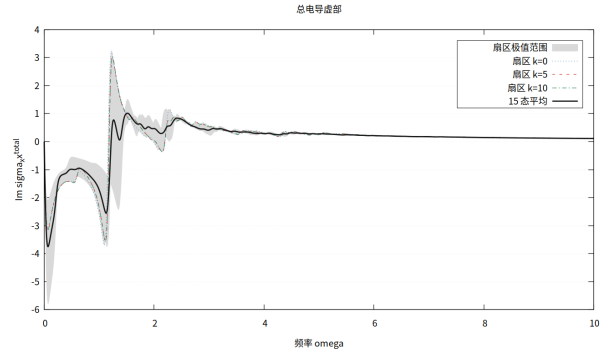
(d) \text{Im } \sigma_{xx}^{\text{total}} : 含 Drude 反应性极点。
