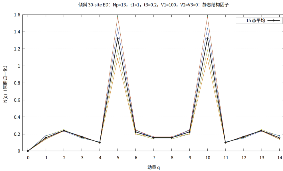
图 13: N_p=13 强耦合候选流形的结构因子。彩色细线是扇区 0:14 各自的 full ED 基态结果，黑色粗线是 15 态等权平均； q = 5, 10 的等高峰是周期三密度序的静态结论，阴影范围表示 1.081443970873–1.579102752688 的扇区差异。
