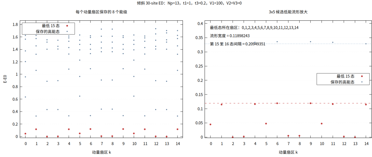
图 12: N_p=13 强耦合参数点的 30-site full ED 能谱。每个扇区由 ED 保存最低 8 个能级，左图显示全能窗，右图放大扇区 0:14 的候选流形；红色标记 15 态，蓝灰色标记更高能级。15 态宽度为 0.11898243171037848，第 15–16 态间隔为 0.20949350939918077，所以图示的低能带确实是有限尺寸的候选流形。
