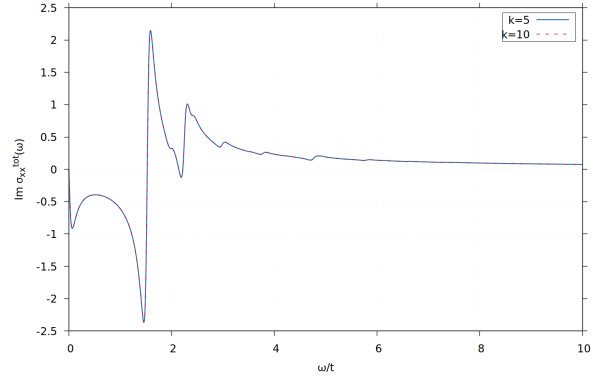
(d) \text{Im } \sigma_{xx}^{\text{total}} .
