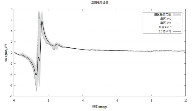
(b) \text{Im } \sigma_{xx}^{\text{reg}} : ED resolvent 色散。
