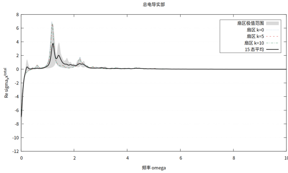
(c) \text{Re } \sigma_{xx}^{\text{total}} : 吸收加 Drude 展宽项。
