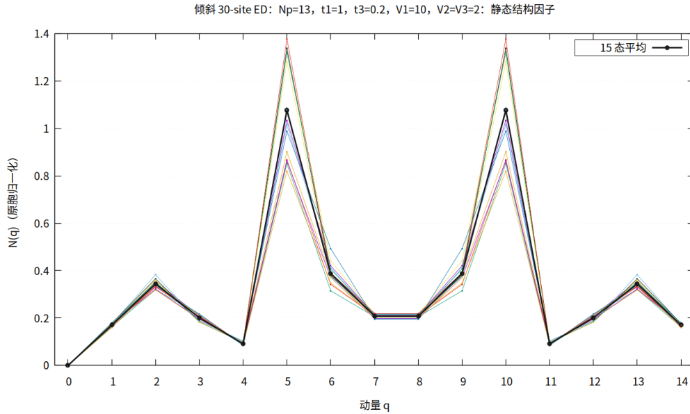
图 16: N_p=13 温和候选流形的结构因子。细线来自扇区 0:14 各自的 full ED 基态，黑线是 15 态等权平均； q=5, 10 主峰及 q=6, 9 次峰分别给出周期三晶体序和其余有限尺寸结构，扇区主峰范围为 0.819697952425–1.376882017093。
