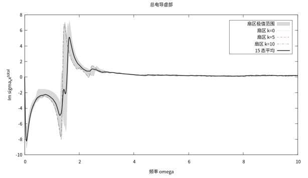
(d) \text{Im } \sigma_{xx}^{\text{total}} : 含反应性 Drude。
