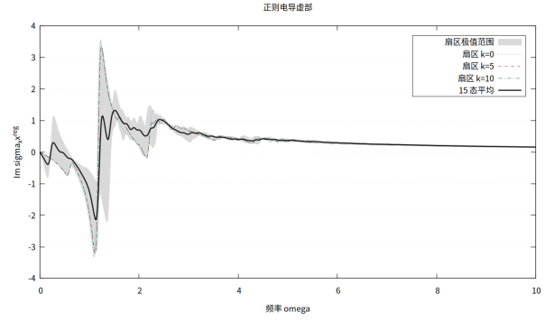
(b) \text{Im } \sigma_{xx}^{\text{reg}} : 同一 ED resolvent 的色散。
