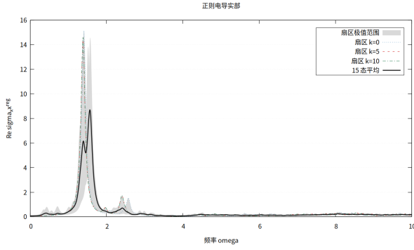
(a) \text{Re } \sigma_{xx}^{\text{reg}} : \eta = 0.065 展宽吸收。
