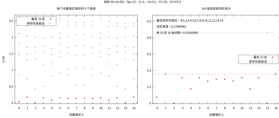
图 15: N_p=13 温和参数点的 30-site full ED 能谱。每个扇区保留 8 个能级，红点标记扇区 0:14 各一态的 15 态候选流形，蓝灰点为其余能级；图中标出的 0.1780098138966082 是流形宽度，0.25265895492933055 是第 15–16 态间隔。
