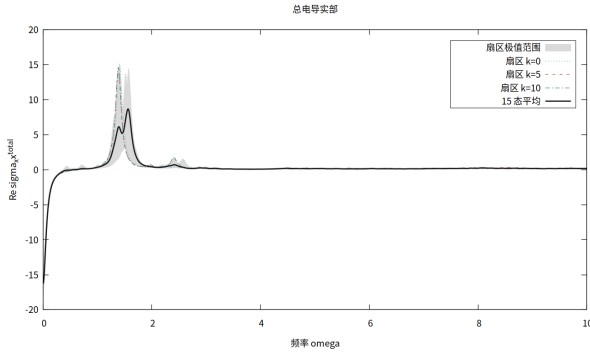
(c) \text{Re } \sigma_{xx}^{\text{total}} : regular 加 Drude。
