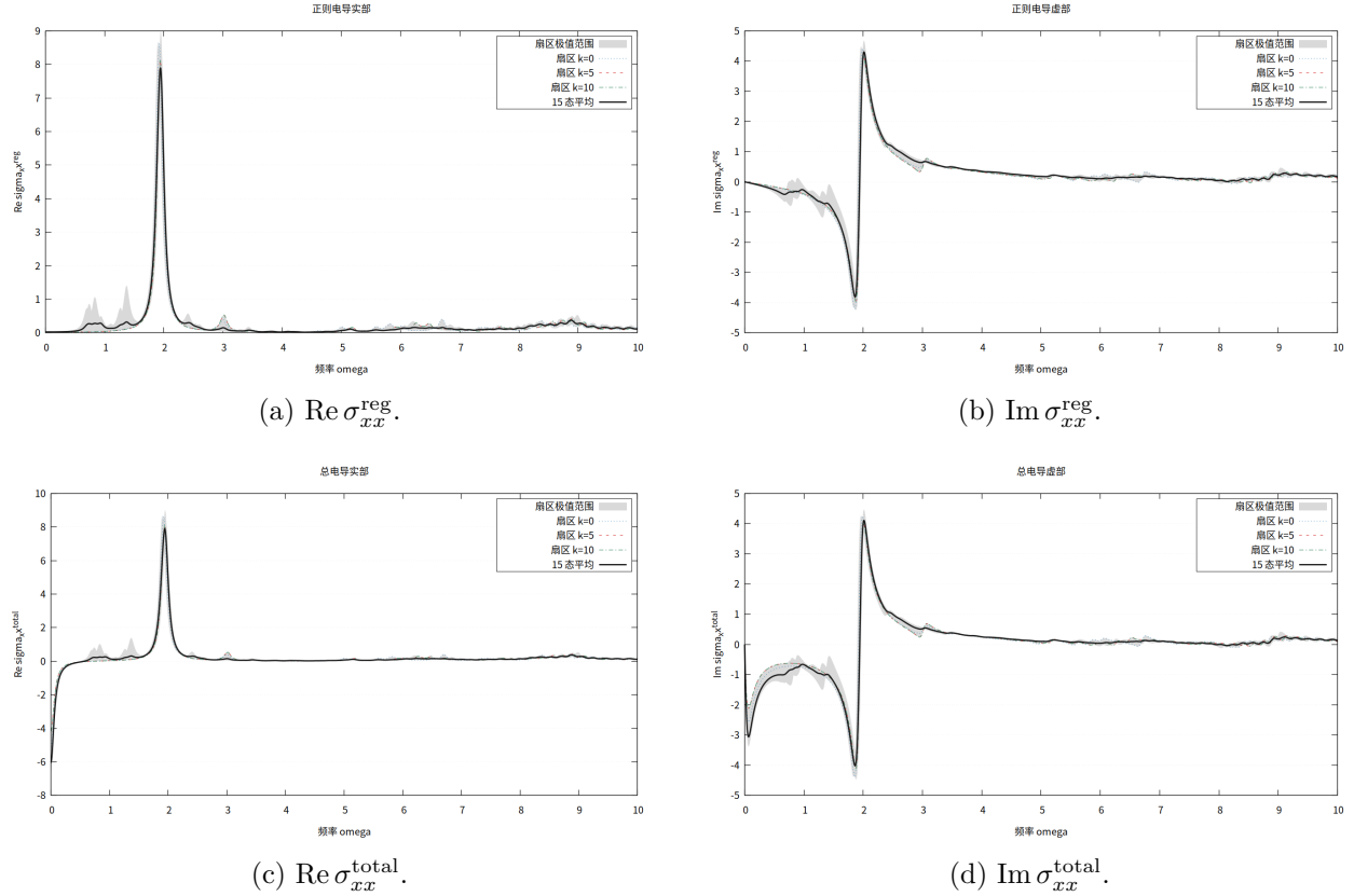
图 11: 温和参数 FQAH 候选流形的纵向光电导。每条单-sector 曲线均由 response-Lanczos ED 独立计算；黑线是 15 态等权平均，灰带给出 sector 间离散。四图使用相同的 M = 600 、 \eta = 0.065 和频率网格。
