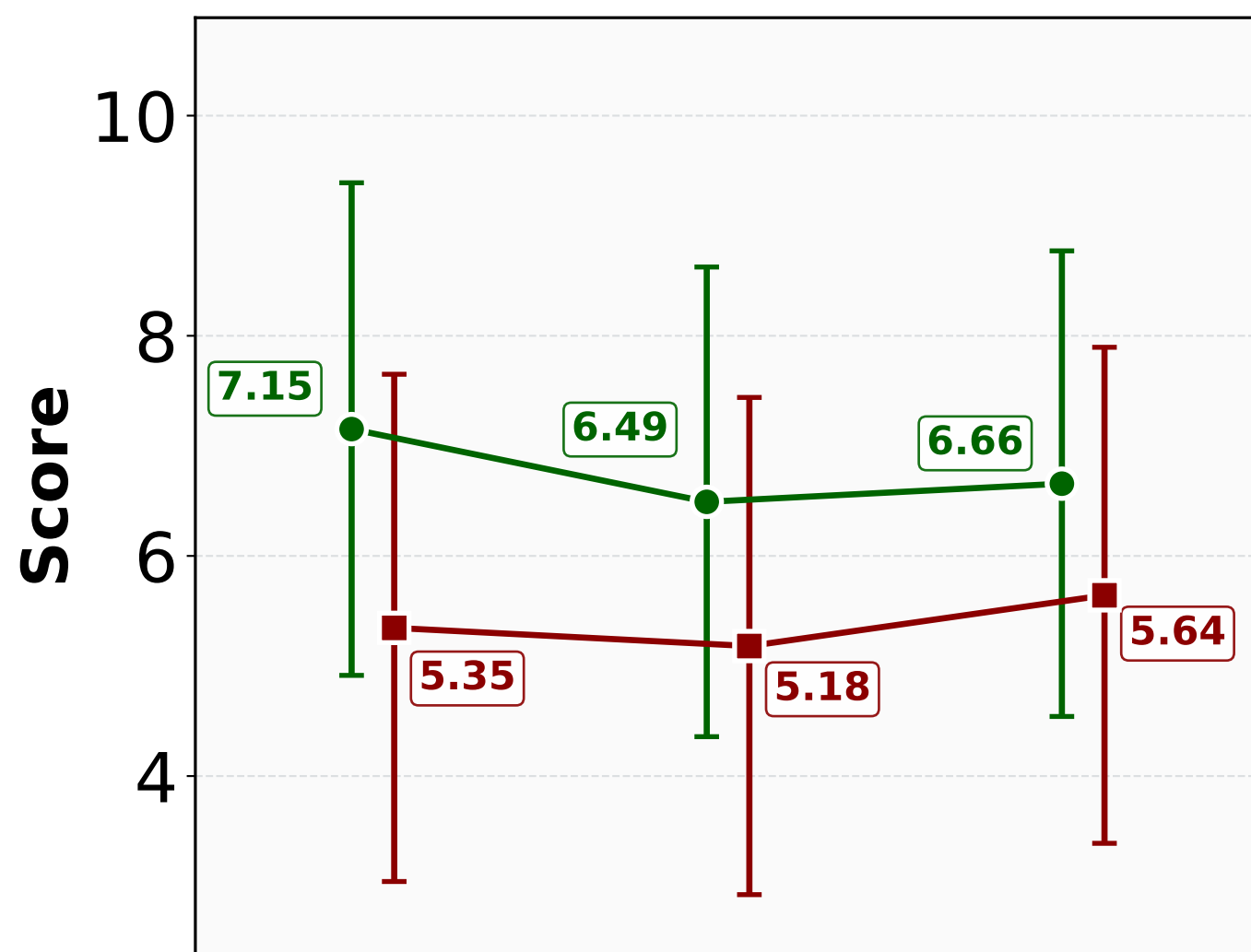
DeepSeek-GRM-16B
