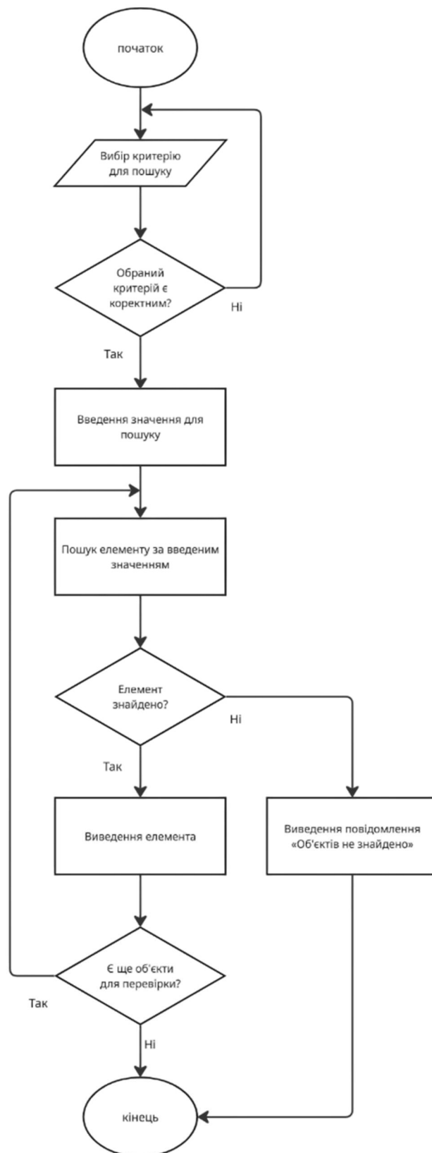
Рисунок 4 – Узагальнена блок-схема алгоритму пошуку та виведення об'єкта
