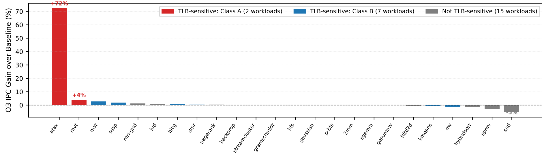
O3 IPC Gain per Workload
