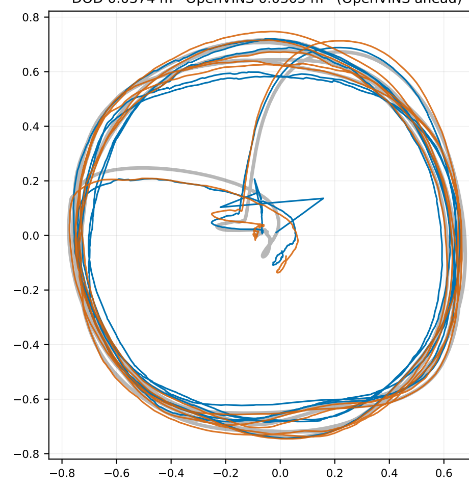
KAIST circle DOD 0.0374 m OpenVINS 0.0305 m (OpenVINS ahead)
