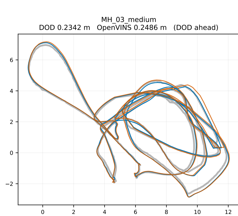
MH_03_medium DOD 0.2342 m OpenVINS 0.2486 m (DOD ahead)
