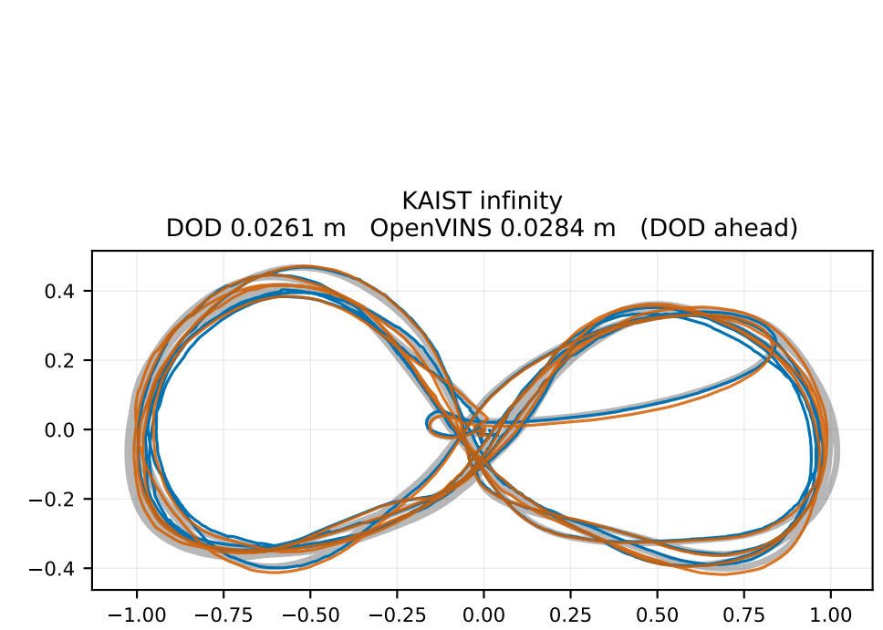
KAIST infinity DOD 0.0261 m OpenVINS 0.0284 m (DOD ahead)
