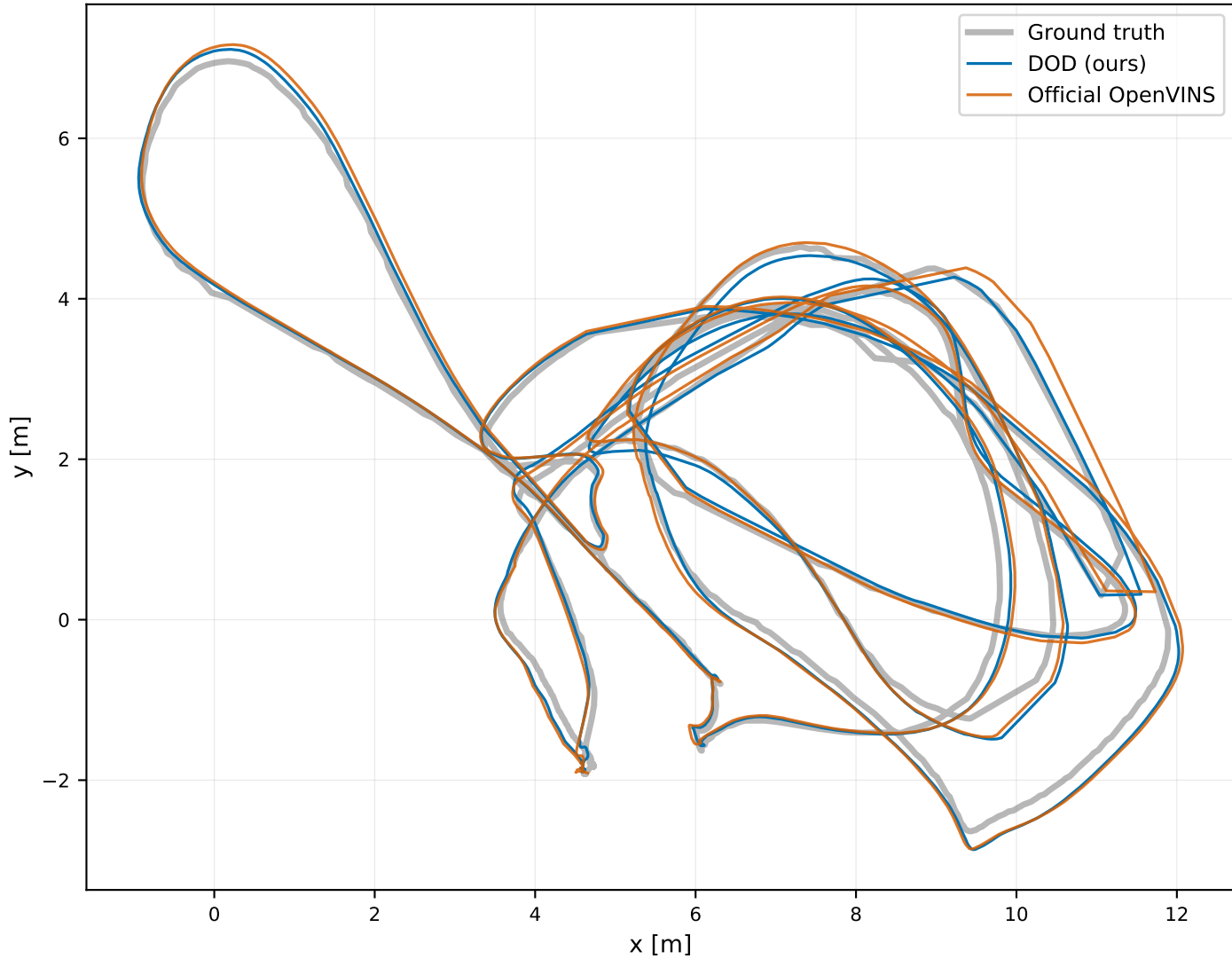
MH_03_medium DOD 0.2342 m OpenVINS 0.2486 m (DOD ahead)
