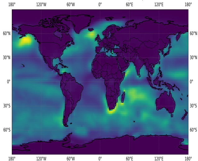
EC-AEREarth3 - Global - DMS Emissions (2xDMS)
