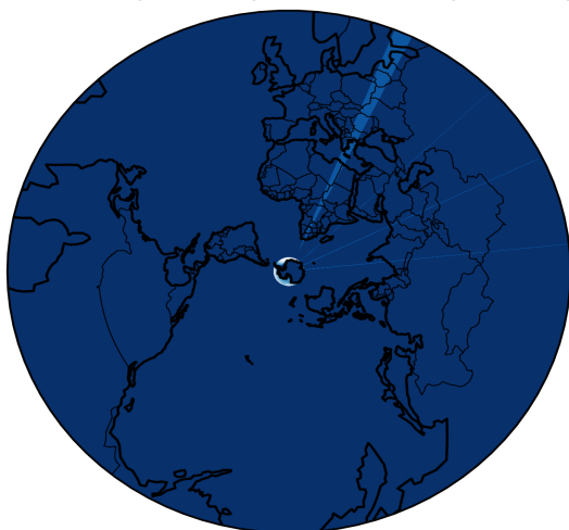
NorESM (control) – Antarctic (control)
