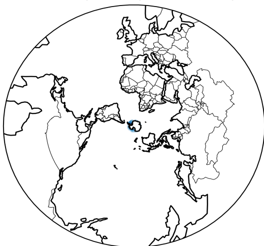
EC-AEREarth3 (control) - Antarctic (control)
