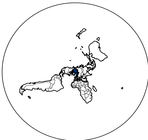
GISS (control) - Arctic (control)
