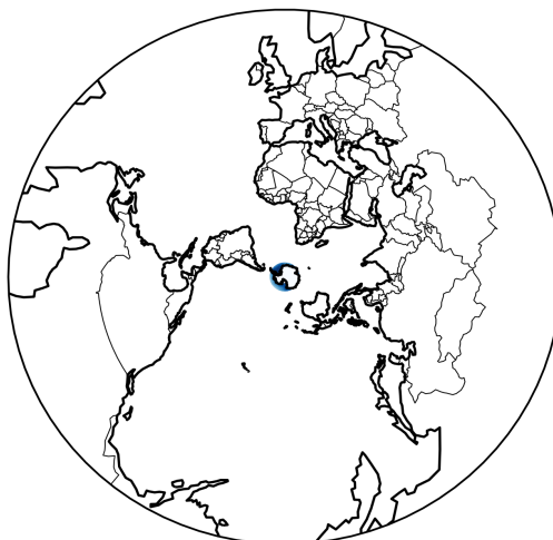
GISS (control) - Antarctic (control)
