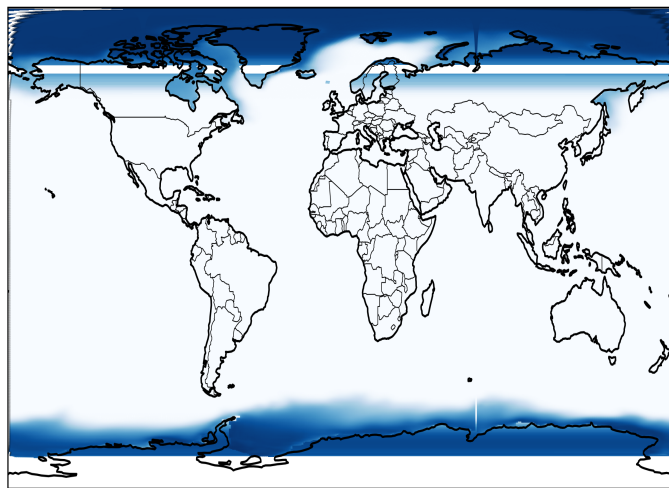
UKESM (control) – Global (control)
