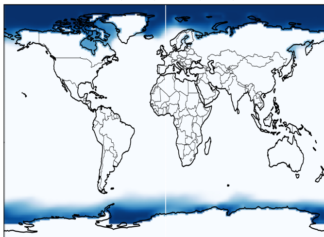
GISS (control) - Global (control)
