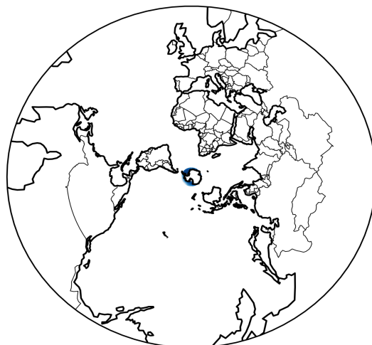
UKESM (control) – Antarctic (control)
