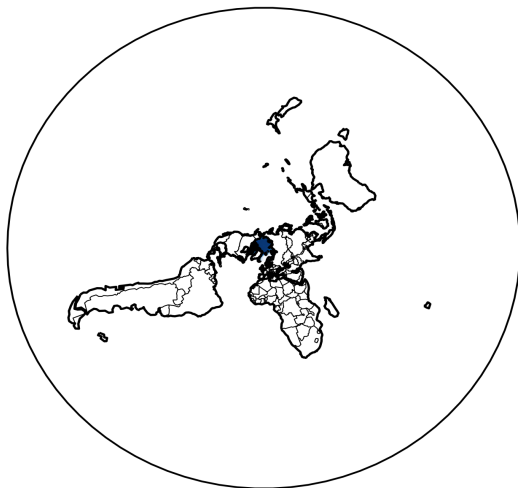
UKESM (control) – Arctic (control)
