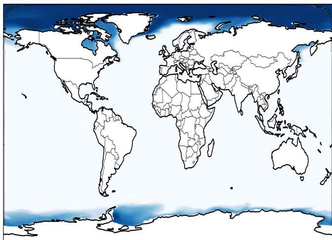
EC-AEREarth3 (control) - Global (control)
