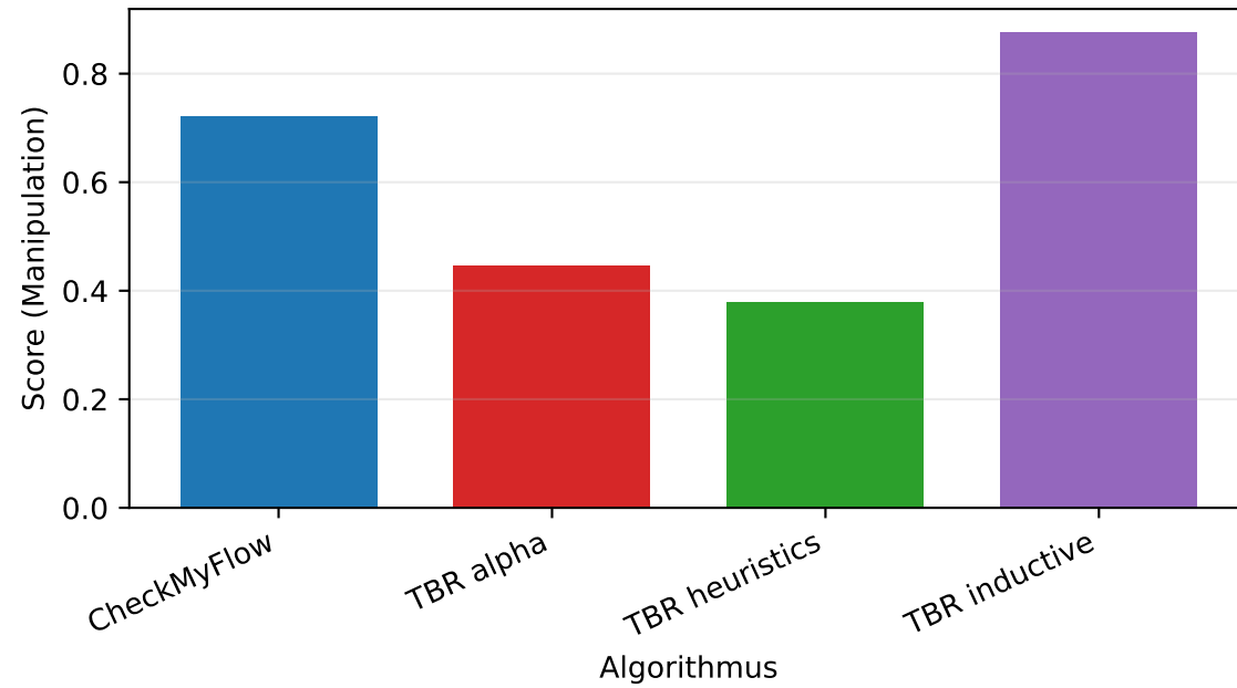
Sepsis
