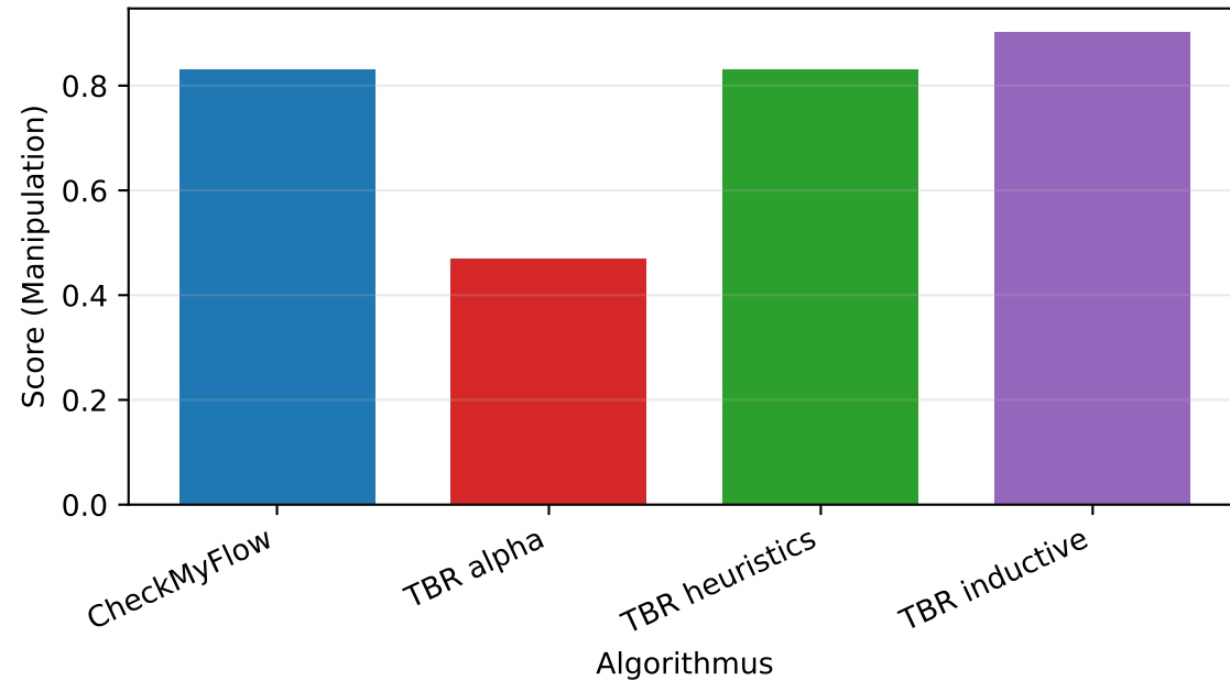
Sepsis
