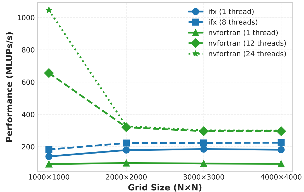
(d) Double Precision - Computational Performance
