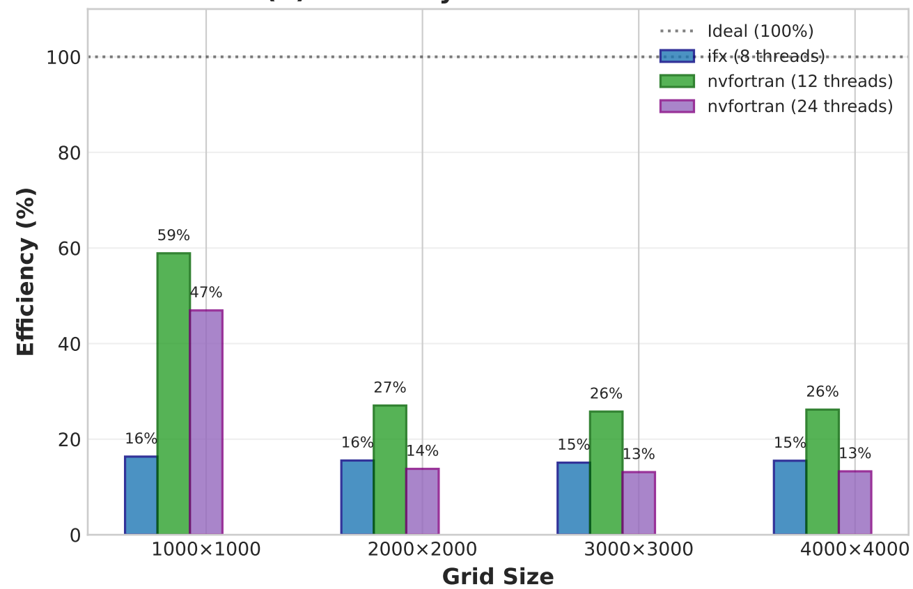
(d) Efficiency - Double Precision
