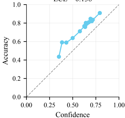
EDL ECE = 0.138
