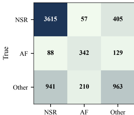
SNGP
