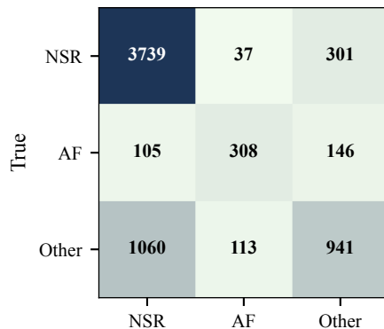
EDL
