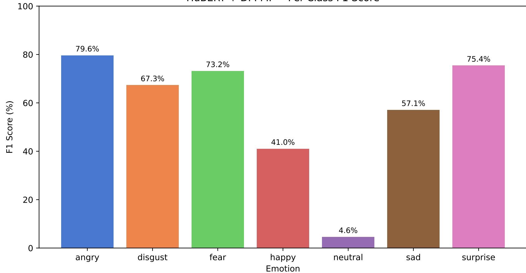
HuBERT + DPPMI — Per-Class F1 Score
