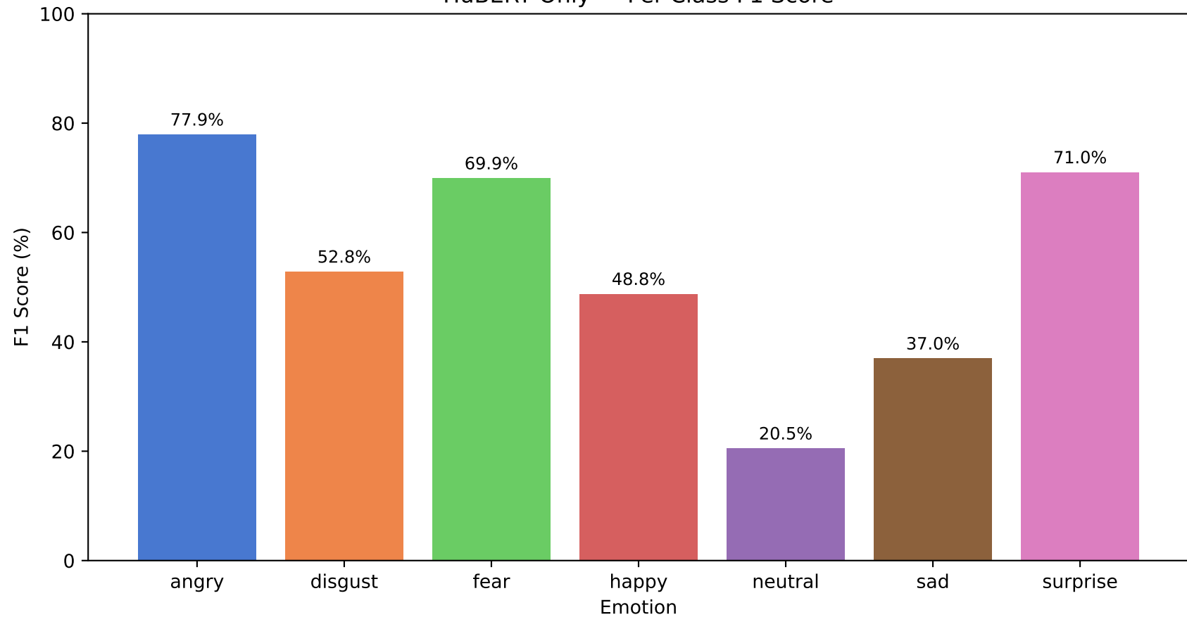
HuBERT Only — Per-Class F1 Score
