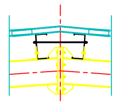
04 TYP. MID FRAME TIE ROD SCALE 1:10
