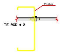
1A SECTION NTS
