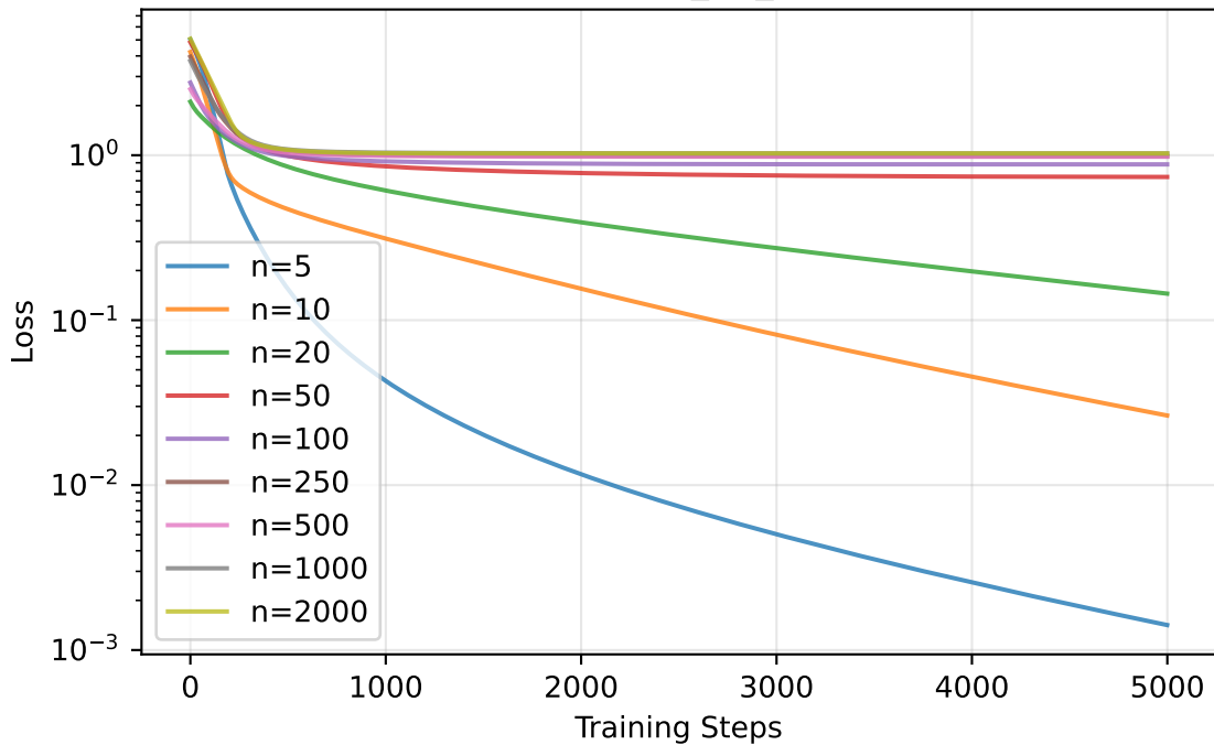
MEDQA: MCal_CE_Uncond
