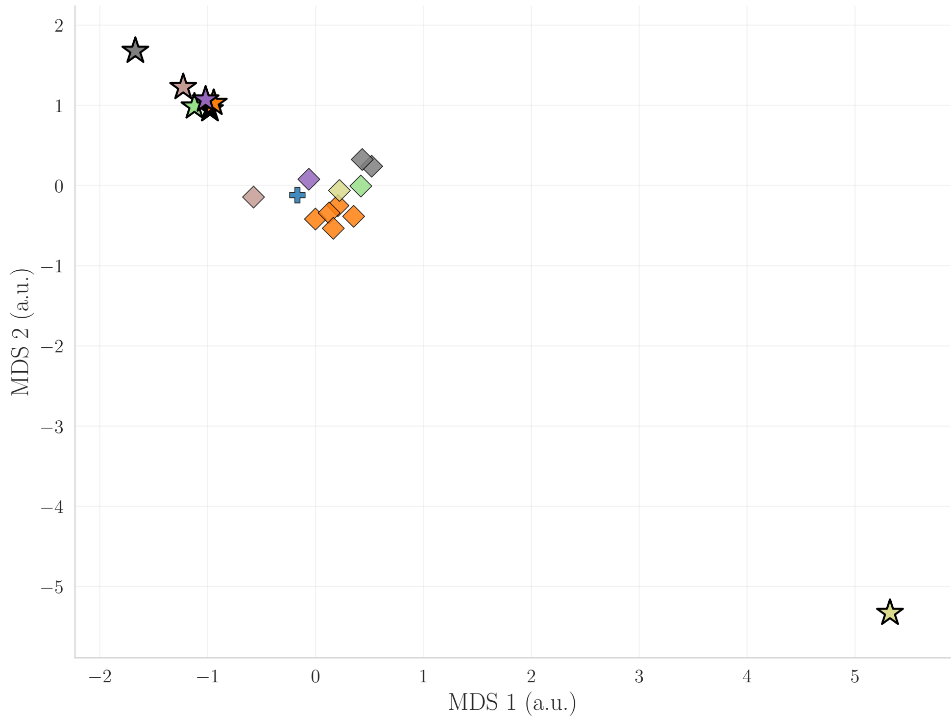
Procrustes MDS (metric)
