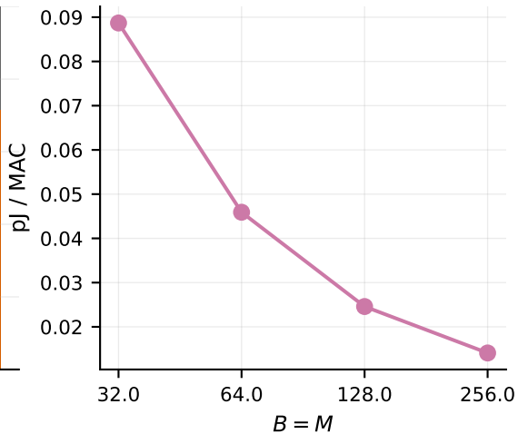
Energy per MAC
