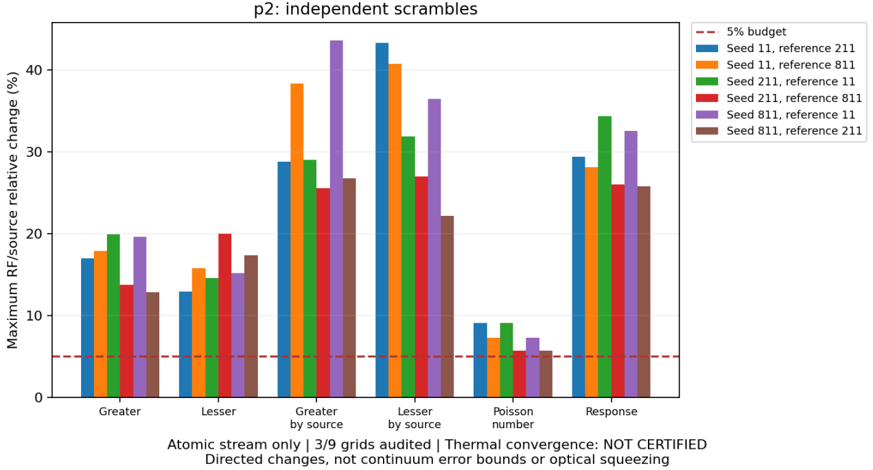
그림 6: 열적 p2 세 scramble의 여섯 유형 비교. 수평 기준선은 5%다. 각 곡선은 같은 물리 조건의 quadrature 표본을 바꾼 결과이며, 다른 실험 detuning·온도·pump 조건에서의 예측 검증을 뜻하지 않는다. 그림과 복소 행렬은 고정된 캠페인 증거를 재사용했다.
