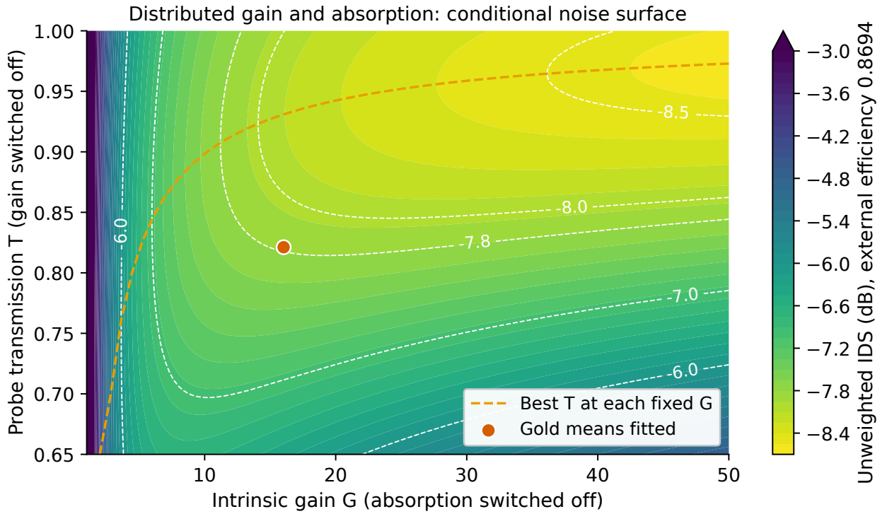
그림 2: 내부 이득과 probe 흡수가 만드는 스퀴징 함수 및 단면. 표시된 이변수 영역의 최소는 이득 상한 경계에 있다. 표 3의 유한 최적점은 고정 흡수 또는 공통계수 변화라는 조건에 의존한다.
