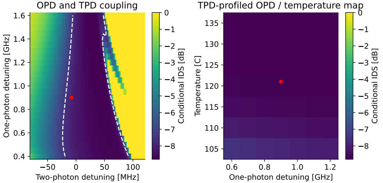
그림 4: Gold 이득을 일계수로 보정한 GABES의 조건부 IDS. 왼쪽 흰 선은 -7.443\text{ dB} 이고, 오른쪽은 TPD를 탐색 구간 안에서 재조정한다. 붉은 점은 gold 기준이다. 잡음은 식 (27)로 환산한다.
