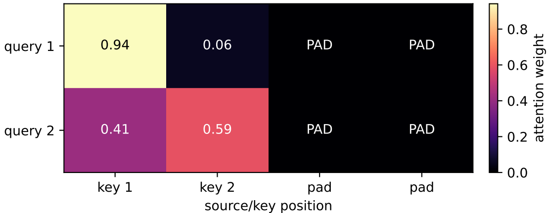
Mask source padding before softmax
