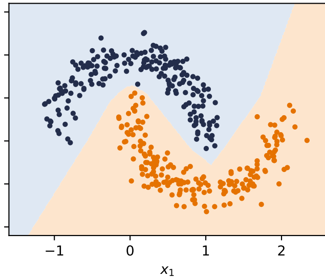
MLP (16 hidden): 100.0%
