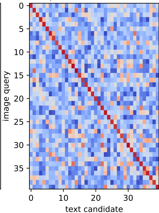
paired · seed 6052
