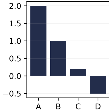
logits o_j
